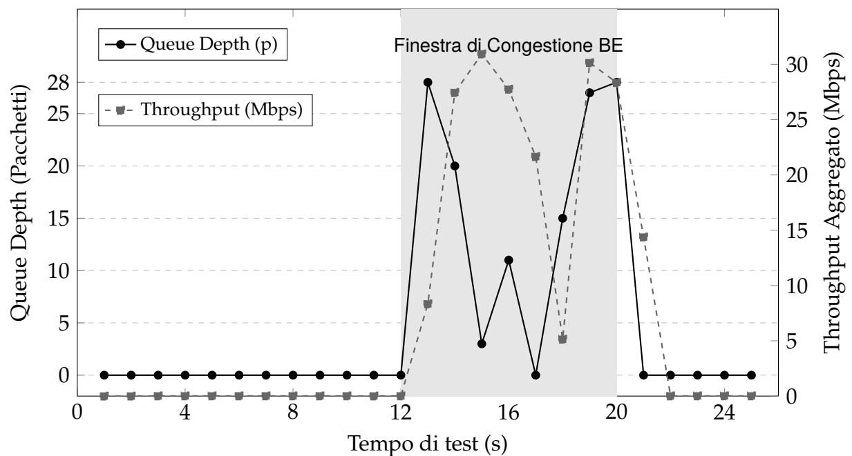
Figura 3.9: Andamento simultaneo della profondità di coda ( Queue Depth ) e del Throughput aggregato nello scenario con TAPRIO, evidenziando l'accumulo nei buffer durante la finestra di congestione.
