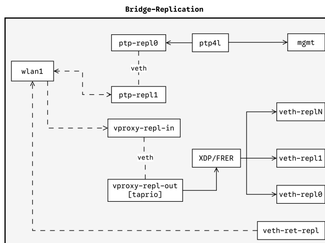
Figura 3.4: Incapsulamento wlan1 per l'utilizzo di ptp4l
