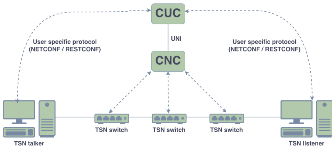
Figura 1.8: Modello Completamente Centralizzato
