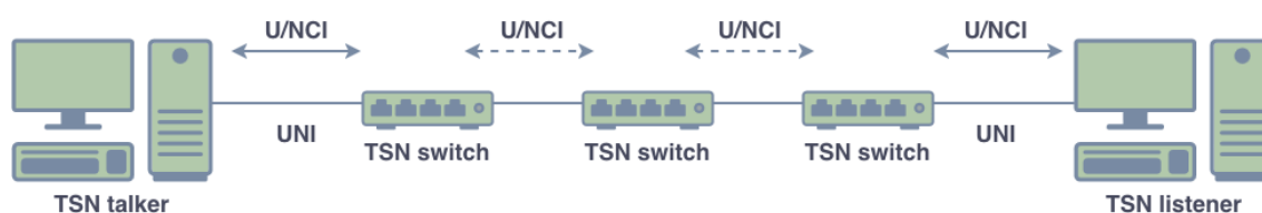
Figura 1.6: Modello Completamente Distribuito
