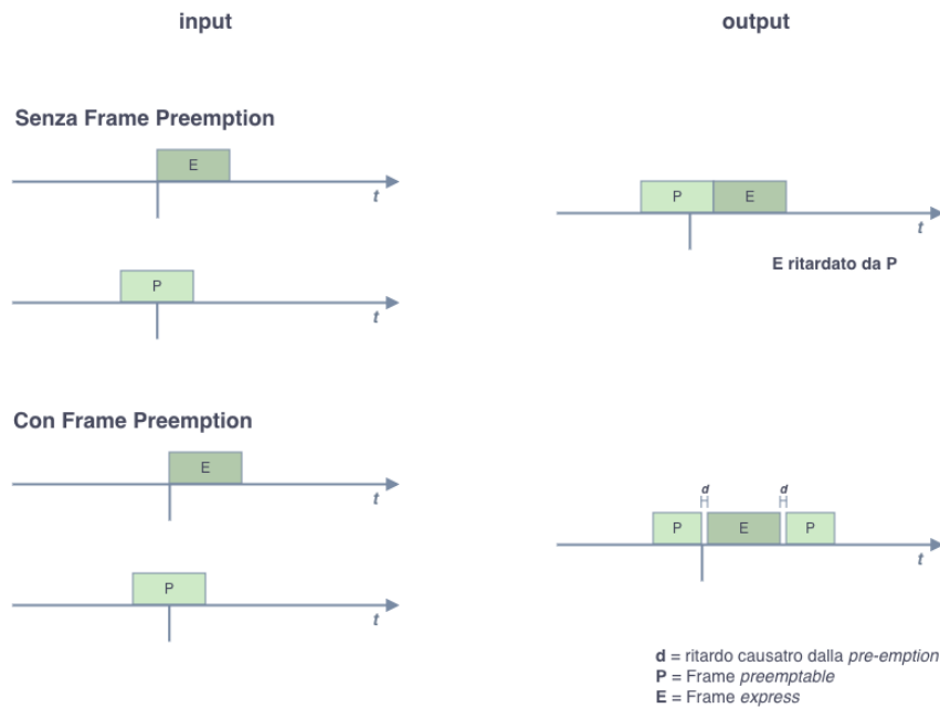
Figura 1.3: Differenza nella gestione del traffico con e senza frame preemption
