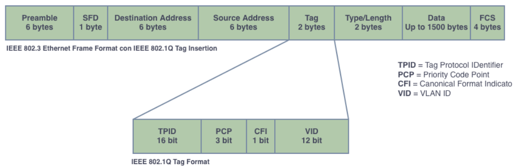
Figura 1.2: IEEE 802.3 Ethernet Frame Format con IEEE 802.1Q Tag Insertion
