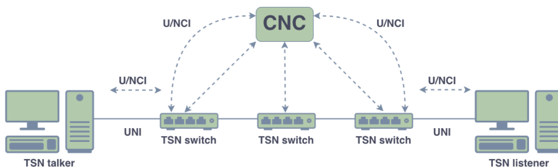
Figura 1.7: Modello a Rete Centralizzata e Utente Distribuito
