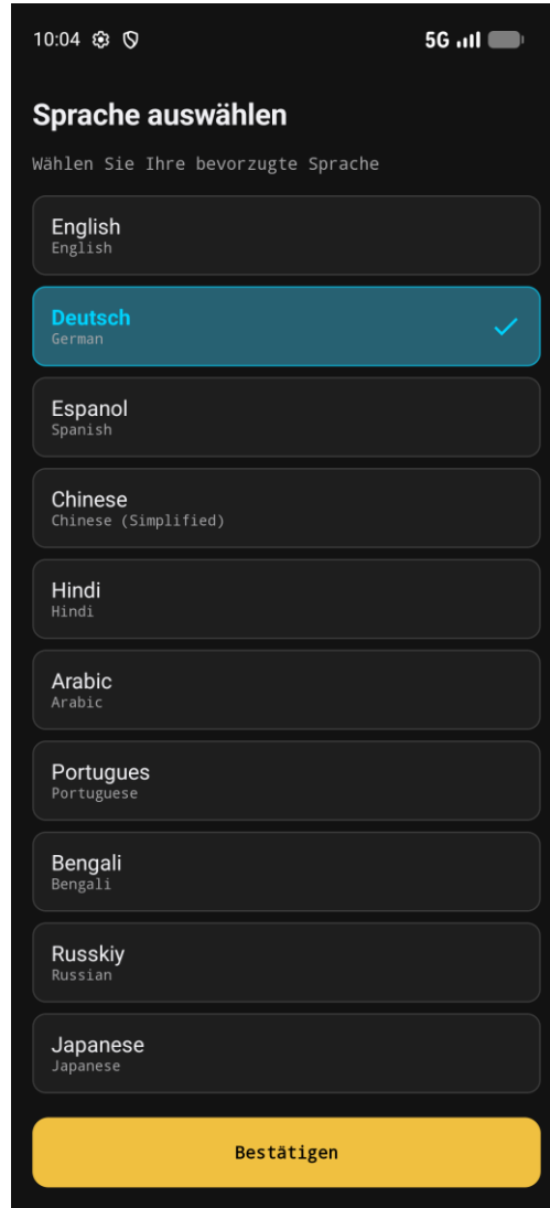
Die Sprachauswahl
