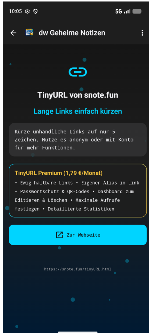
Der TinyURL-Bildschirm
