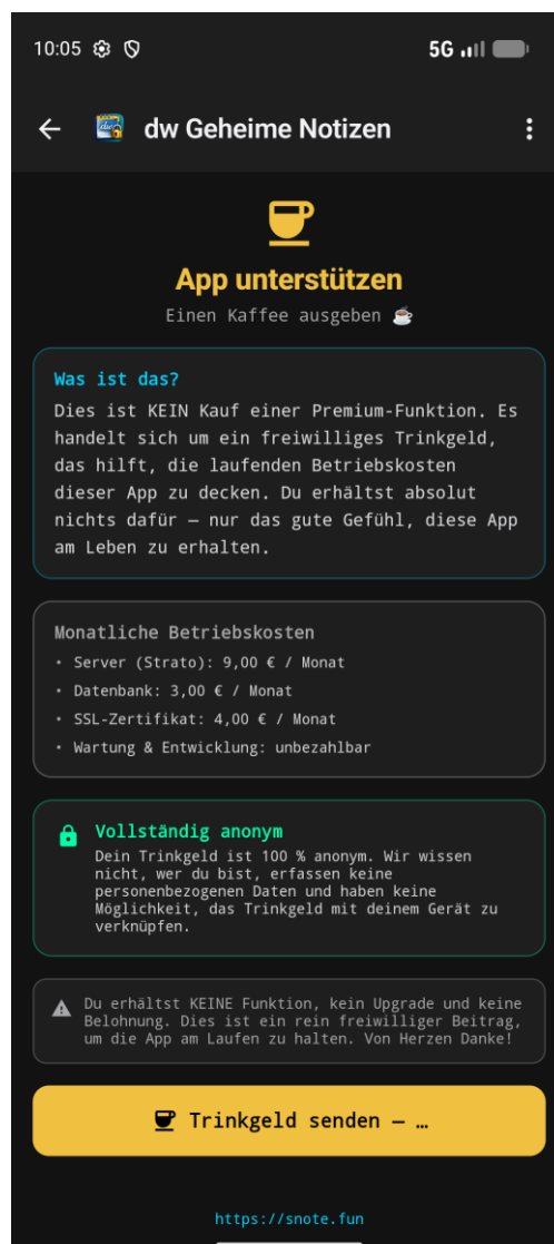
Der Support-Bildschirm
