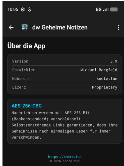
Der Über-die-App-Bildschirm
