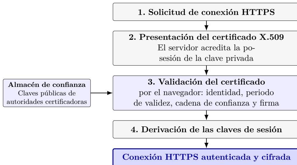
Figura 6: Esquema simplificado del establecimiento de una conexión TLS. Elaboración propia a partir de RFC 8446 [Rescorla, 2018].
