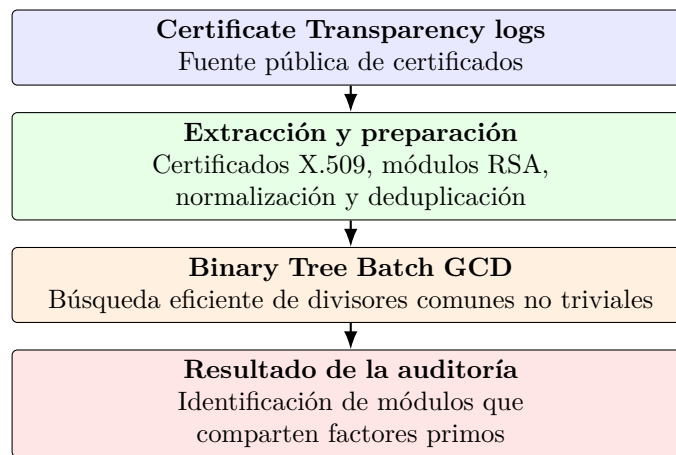
Figura 2: Visión global del problema y del flujo seguido en el TFM.
