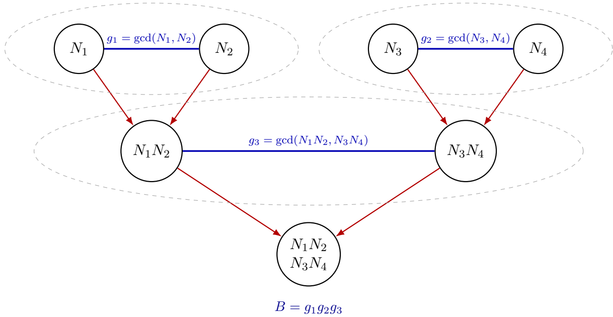
Figura 8: Construcción del árbol en Binary Tree Batch GCD . En cada agrupación se calcula el producto que asciende al siguiente nivel y el GCD entre las dos ramas, cuyos valores no triviales se agregan en B .
