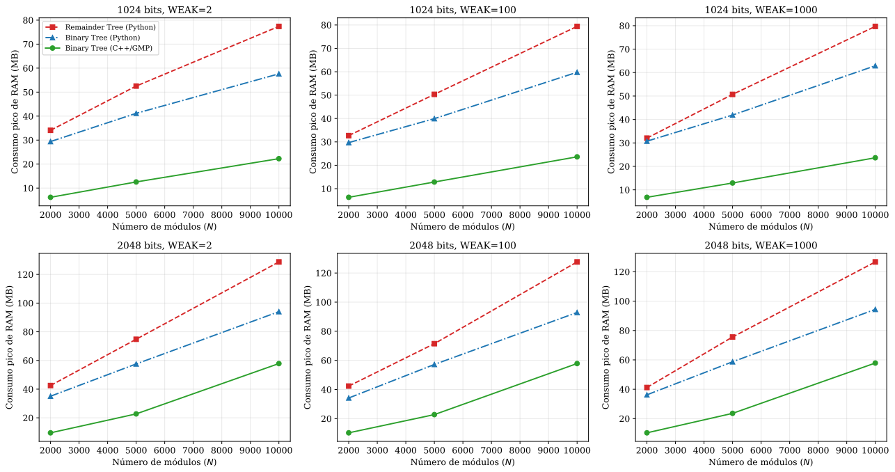
Figura 12: Comparación del consumo pico de memoria de los tres algoritmos evaluados.
