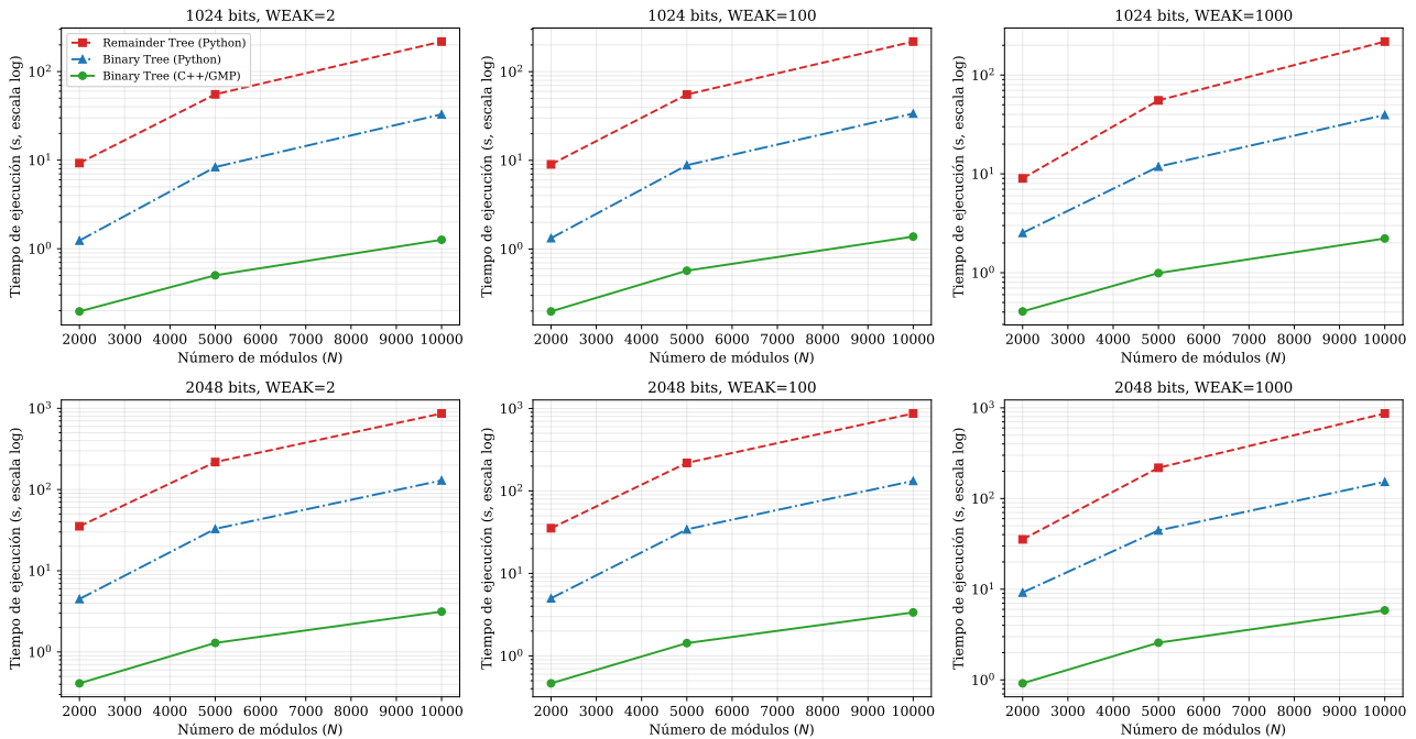
Figura 11: Comparación del tiempo de ejecución de los tres algoritmos evaluados sobre datos sintéticos.
