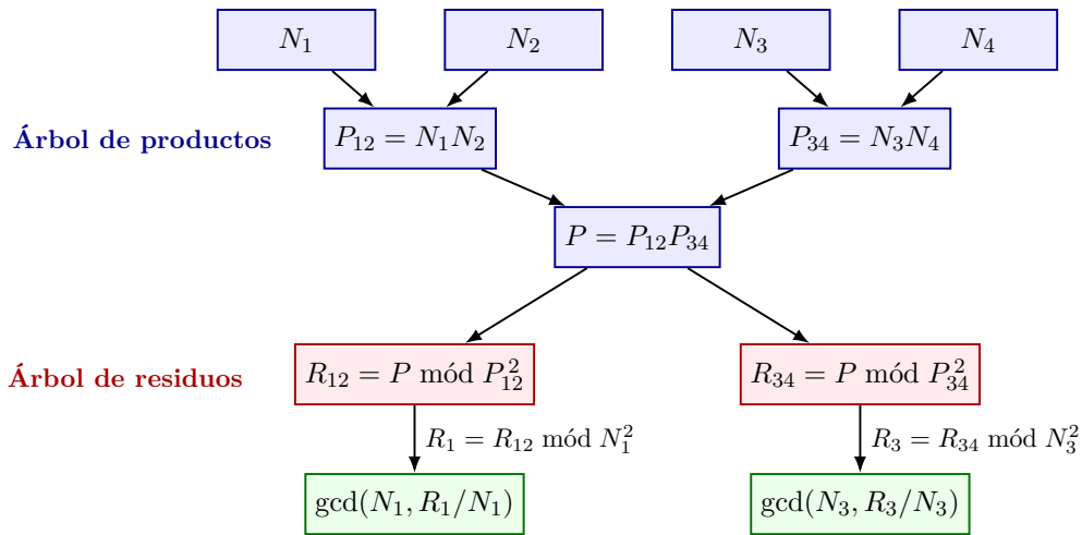
Figura 7: Esquema simplificado del método clásico basado en un árbol de productos y un árbol de residuos. Solo se muestran dos de las cuatro comprobaciones finales para mantener legible la figura.
