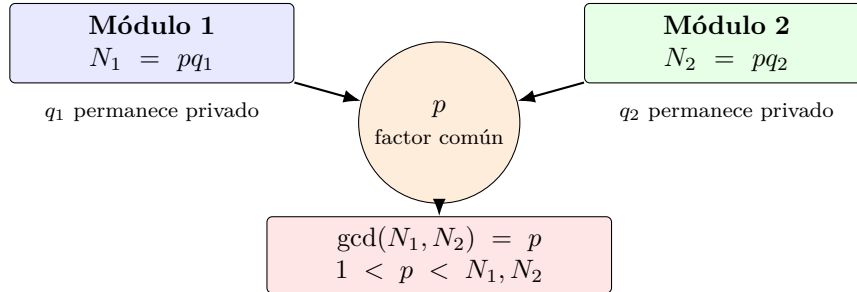
Figura 6: Ejemplo de dos módulos RSA que comparten un factor primo. El cálculo del GCD revela directamente dicho factor.
