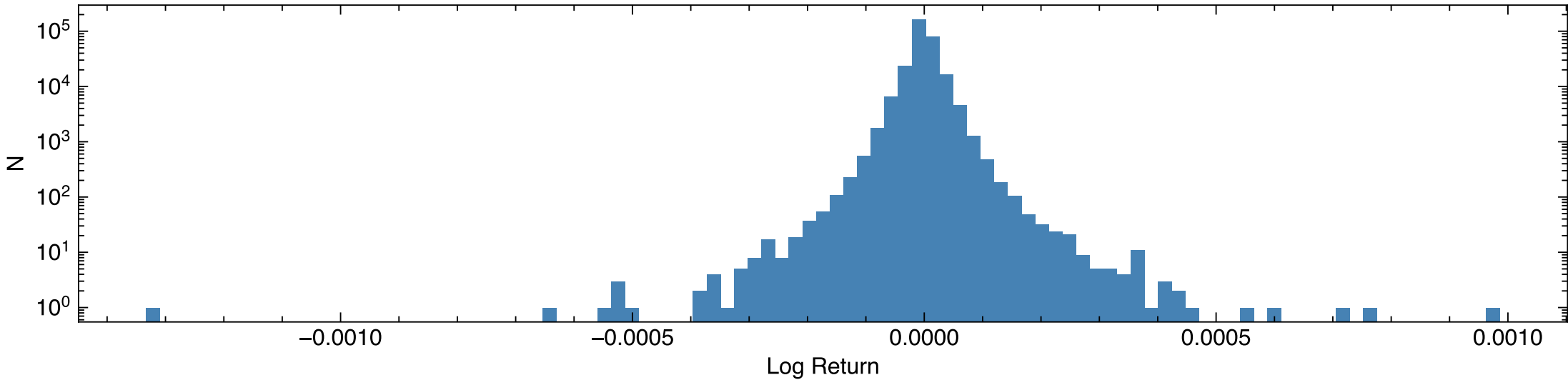
Log Returns
