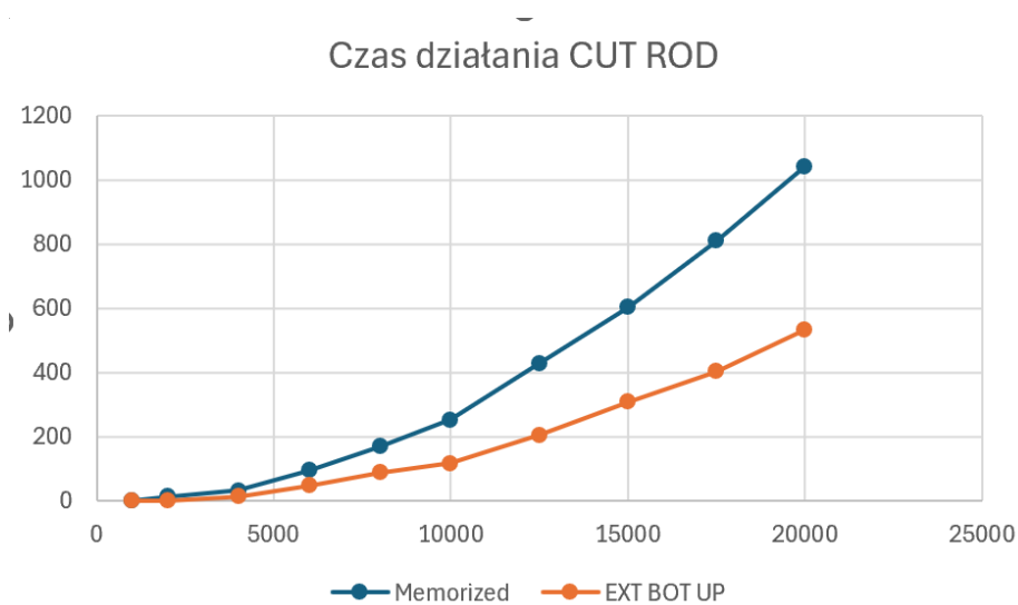
Rysunek 3: Wykres czasu działania algorytmu CUT ROD w wersji ze spamiętywaniem oraz iteracyjną.
