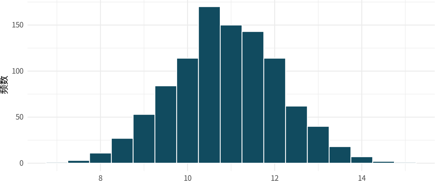
基于自助数据拟合模型的斜率
