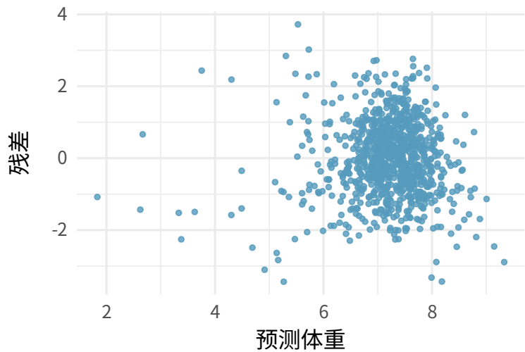
残差 vs. 预测值
