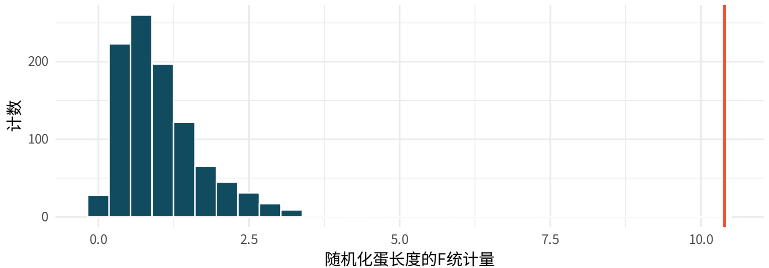
1000个随机化的F统计量
