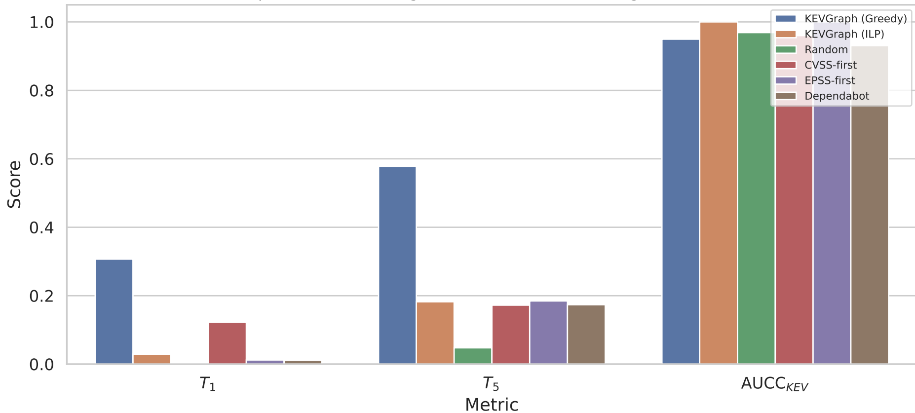
Plan Comparison ( T_1 , T_5 : higher=better; AUCC_{KEV} : higher=faster KEV fix)
