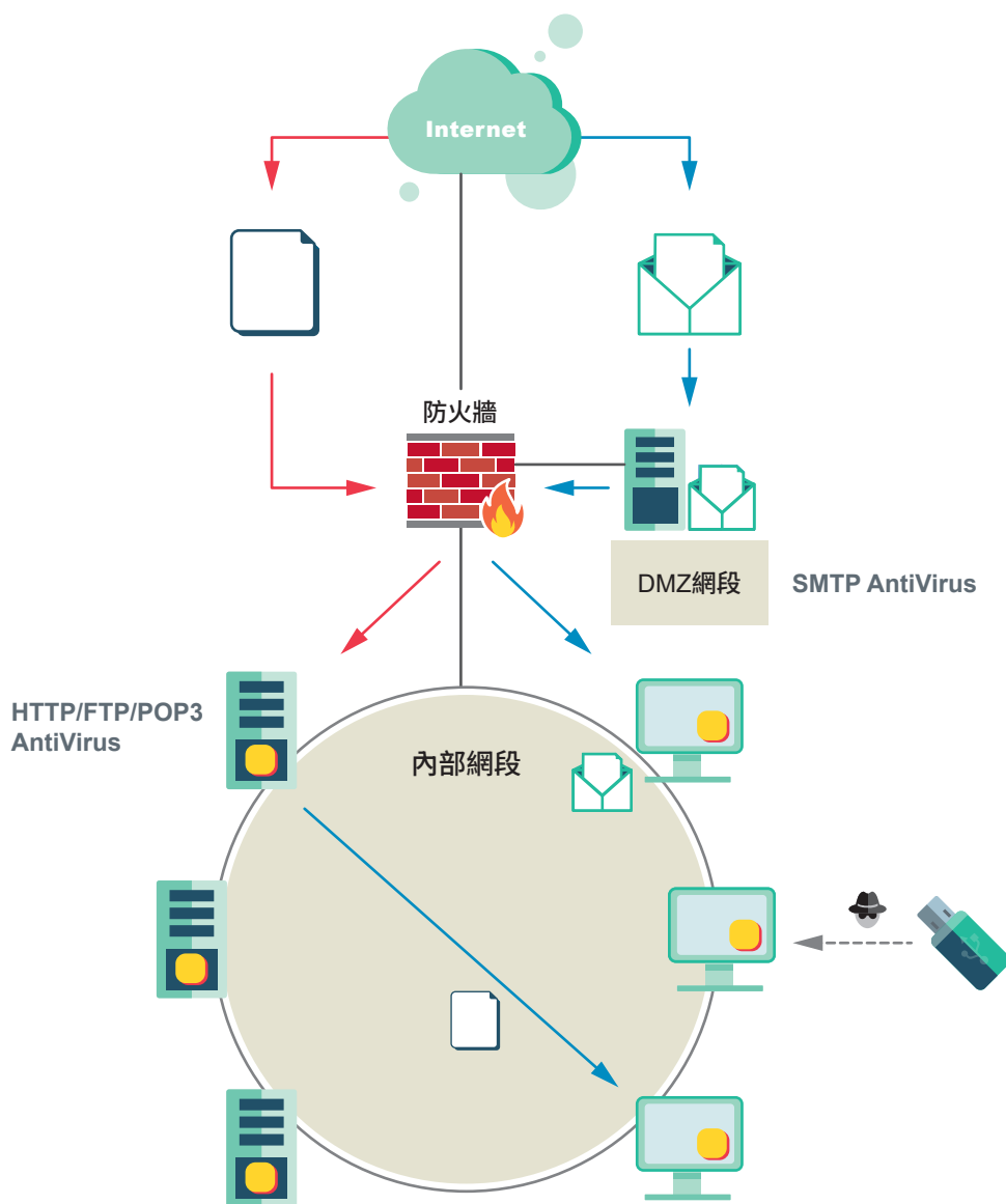
圖40 防毒軟體部署方式示意圖
