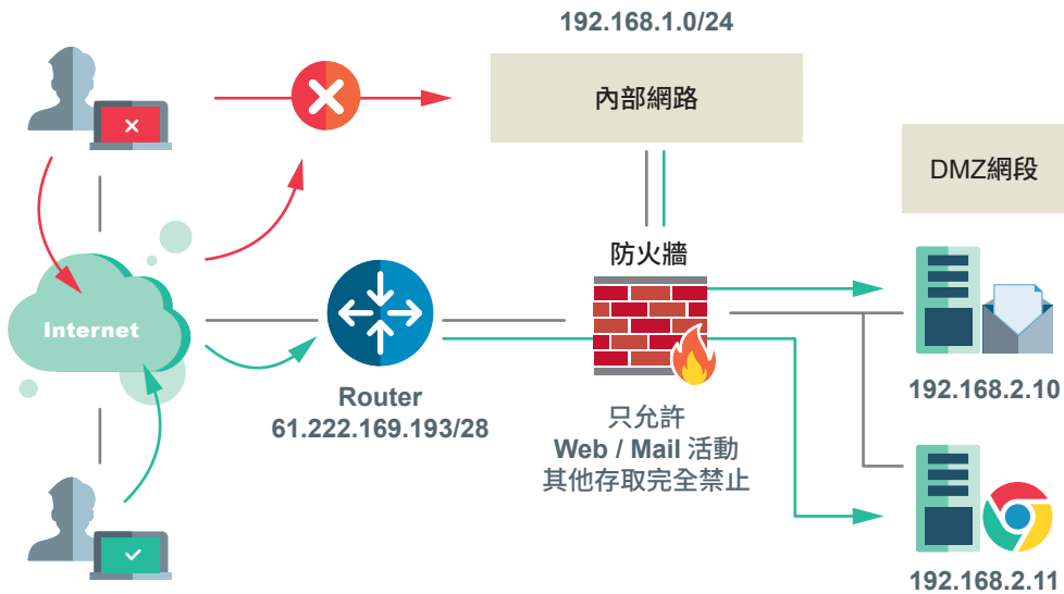
圖41 網路防火牆部署範例
