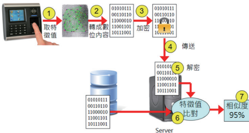
圖30 生物特徵鑑別步驟流程圖
