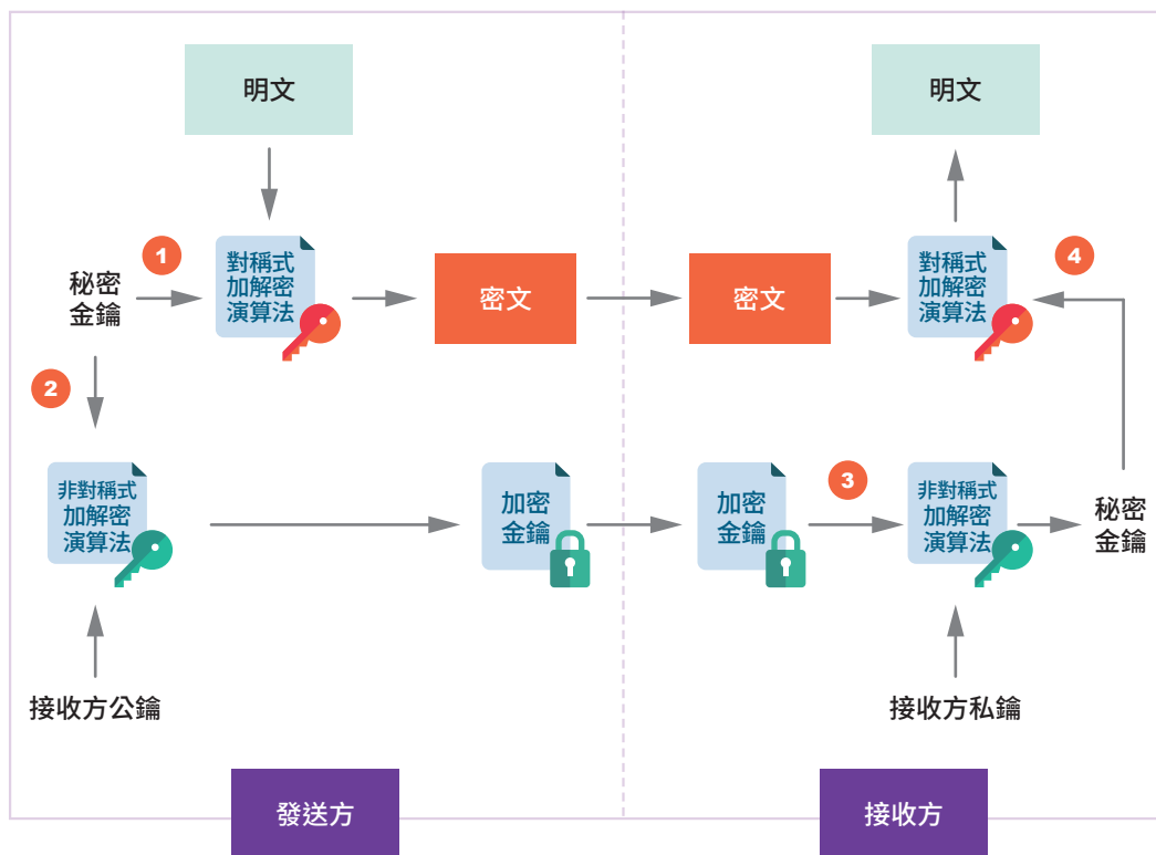
圖37 數位信封運作流程圖
