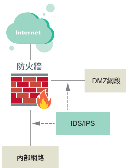
圖48 IDS/IPS設備部署位置示意圖
