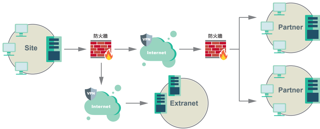
圖60 Extranet VPN示意圖
