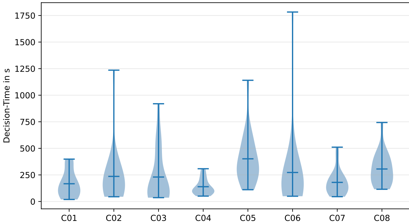
Decision-Time-Verteilung pro Case
