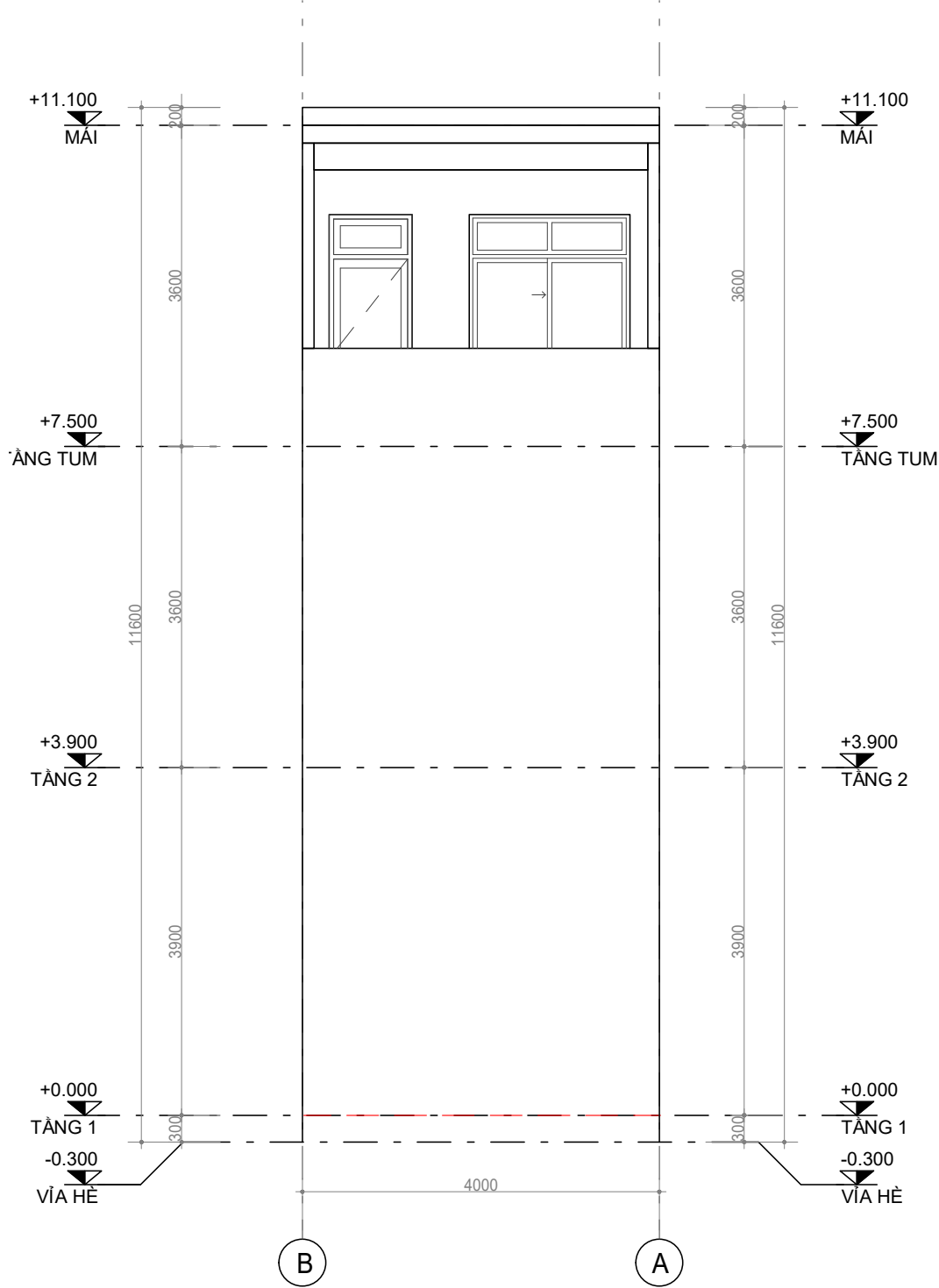
1 MẶT ĐỨNG TRỤC A-B, B-A A2.01 1 : 75
