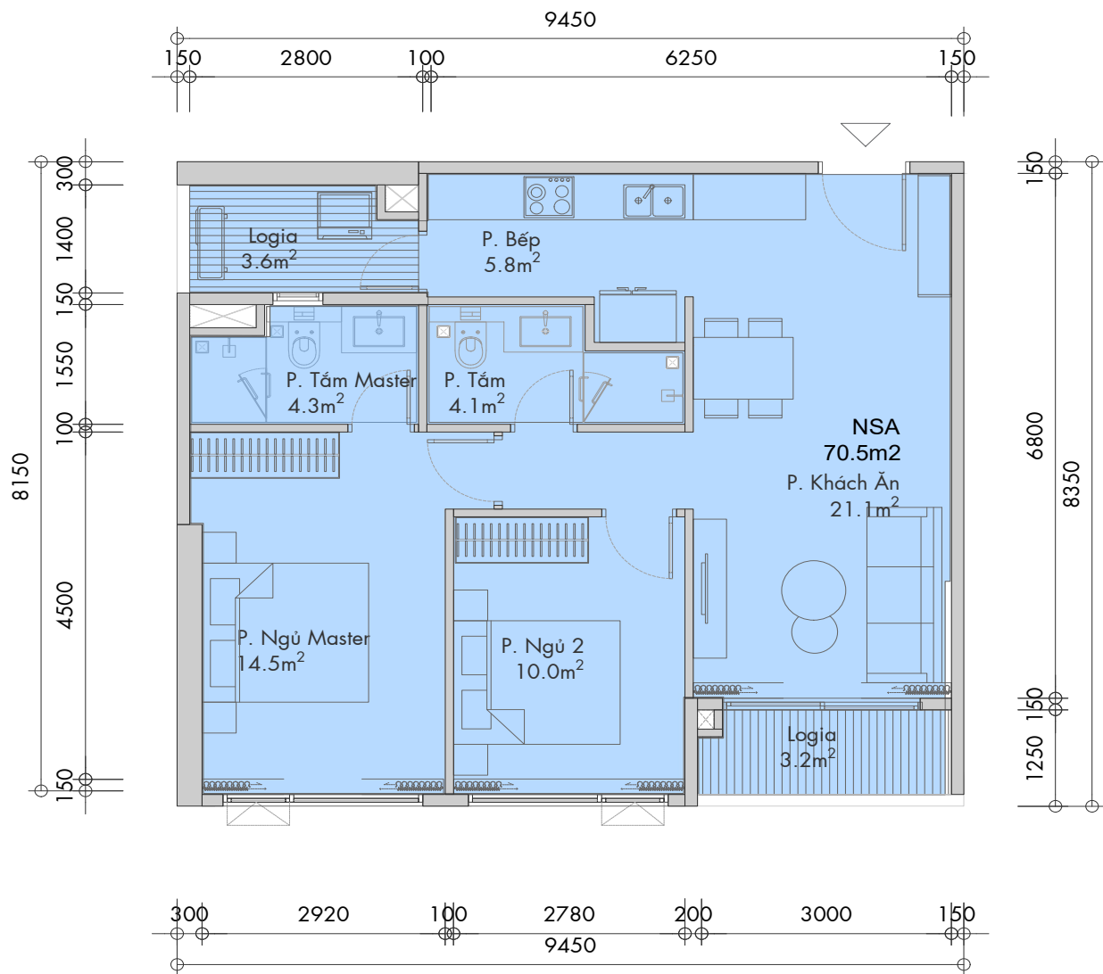
CH-B2 | PHƯƠNG ÁN ĐỀ XUẤT Diện tích sử dụng: 70.5m 2 Diện tích tim tường: 77.5m 2
