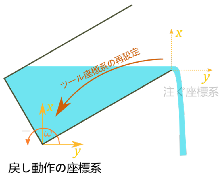
図 2.3: 戻し動作の説明
