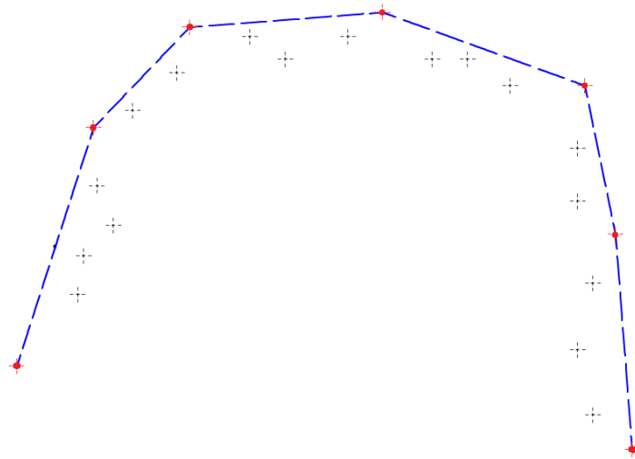
図 4.2: ConvexHull の結果
