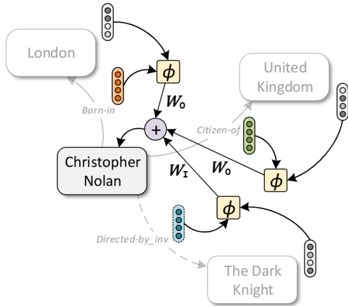
CompGCN Update
