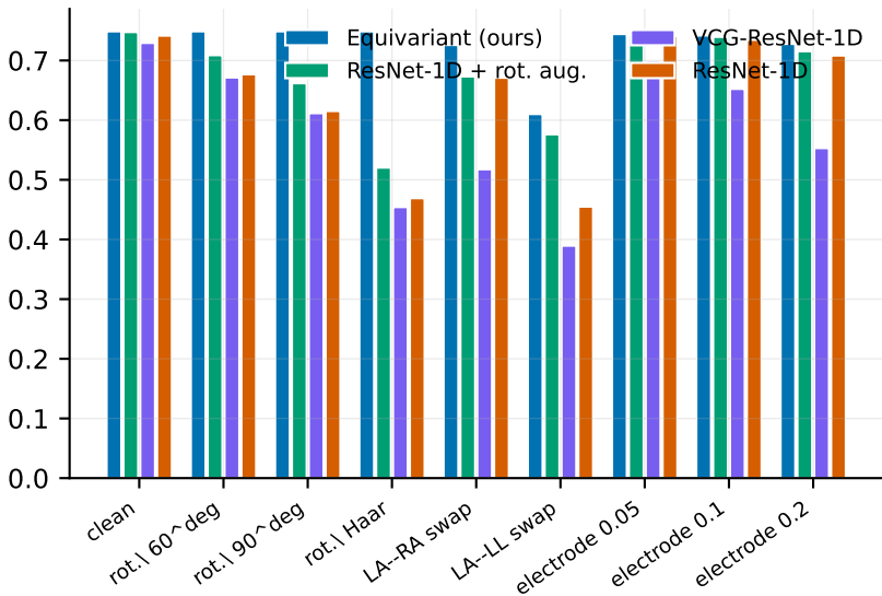
test macro-F1
