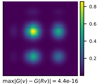
(d) Gram matrix (invariant)
