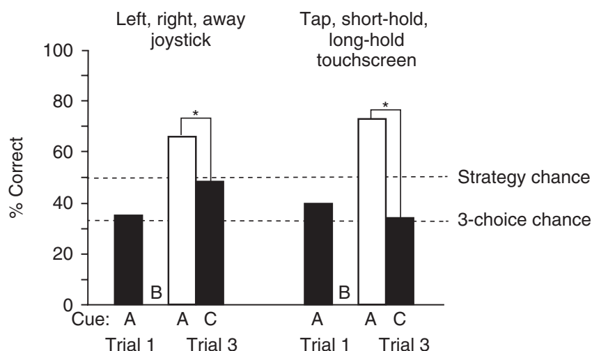
图 8.5: 条件性视觉运动任务中一次试验学习显著。显示了两组数据：一组是三项选择任务，其中猴子必须向不同方向移动操纵杆；另一组是三项选择任务，其中猴子必须点击触摸屏或将手放在屏幕上一段时间。每组三条柱状图显示集合 [A、B、C] 中新刺激的数据。在第一次试验中，猴子的表现符合预期，处于随机水平。然后，纠正程序迫使它们在“试验”结束前选择正确的响应。在第二次试验中，另一种刺激介入，在本例中为刺激 B，表现有时会受到策略效应的影响。第三次试验提供了一次试验学习的测试，与策略效应无关。黑柱状图显示刺激的第一次呈现，白柱状图显示第二次呈现。与刺激 C 第一次出现相比，猴子在刺激 A 第二次出现时表现出明显更好的表现（星号）。对于自发采用换班策略的猴子（左图），正确率有 50%；对于没有采用换班策略的猴子（右图），正确率有 33% [615-616] 。
