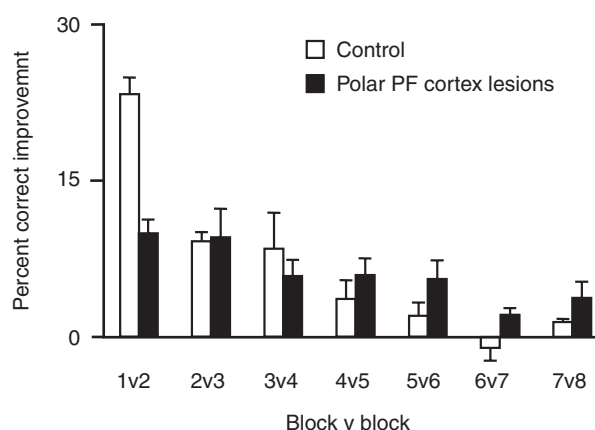
图 3.10: 额极皮层（区域 10）损伤后，第二次试验的物体原位场景任务损伤。每个条形图显示了正常（对照）猴子（白色）和病变猴子（黑色）连续试验块的正确选择百分比的差异。每个选项在 20 个选项的“块”中出现一次。缩写：v，相对于。数据来自 Piekema 等人（2009 年），由 Mark J. Buckley 博士提供。
