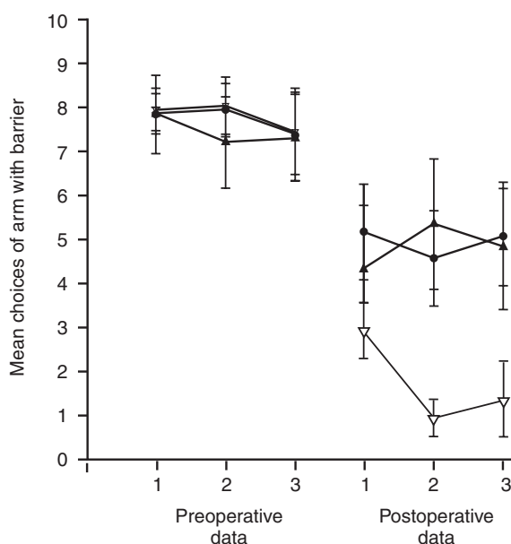
图 3.7: 努力成本对老鼠目标选择的影响。三组老鼠在迷宫的两臂之间进行选择。一只手臂有少量奖励，没有障碍物；另一只获得了巨大的奖励，并且有一个 30 厘米高的障碍，老鼠需要克服这个障碍。纵坐标显示了老鼠在 10 次试验中选择高强度手臂的平均次数。术后，前扣带皮层损伤（未填充三角形）的大鼠选择高强度杆的频率明显低于其他两组：假损伤（填充圆形）的大白鼠和边缘前皮层+边缘下皮层损伤（填充三角形）。误差条：SEM。横坐标上的 1、2 和 3 显示了 3 天的测试数据，每个测试 10 次。转载自 Walton ME、Bannerman DM、Alterescu K、Rushworth MF。前扣带内侧额叶皮层内评估努力相关决策的功能专门化，《神经科学杂志》23:6475-9© 神经科学学会，2003 年，经许可。
