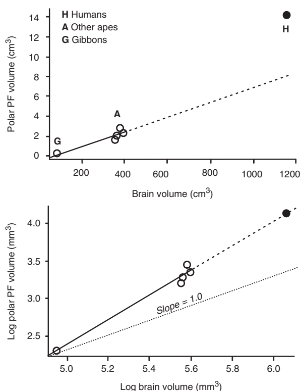
图 9.2: 在选定的灵长类动物群体中，额极皮层体积的回归作为脑体积的函数。实线：来自猿类数据的回归；虚线：外推到人类大脑的大小。顶部：线性刻度。底部：对数刻度，单位斜率由虚线表示。缩写：G，长臂猿；A，类人猿；哈，人类 [663] 。
