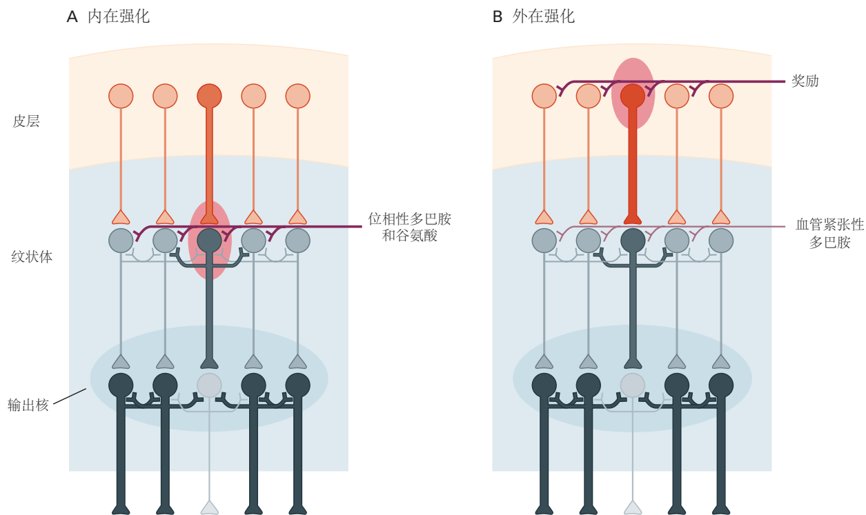
图 38.7.1: 2 个独立的强化机制可以在基底神经节的可重入并行循环结构中进行偏向选择（为清楚起见，省略了通过丘脑的回路返回连接）。 A. 内在强化 （红色椭圆形）涉及皮层纹状体神经传递的选择性敏化（由不同通道中纹状体投射神经元的相对厚度表示）。最近活跃（选定）通道中的传输通过多巴胺和谷氨酸的联合相位性释放得到加强，该释放是由意外的生物学显著感觉事件（例如奖励）引起的。非活动通道缺乏突触多巴胺强化所需的资格迹。由此产生的选择可塑性将导致优先重新选择近期行为输出的强化版本，从而在行动和结果之间建立关联。 B. 最近的研究表明，与奖励（红色椭圆形）的关联可以加强向纹状体提供传入信号结构中的处理。就基底神经节的选择部分取决于输入到纹状体信号的相对强度（广泛接受的观点），与奖赏相关的传入信号调节实际上会选择偏向于奖励相关的输入。同样，图中投射的粗细表示激活的相对水平。
