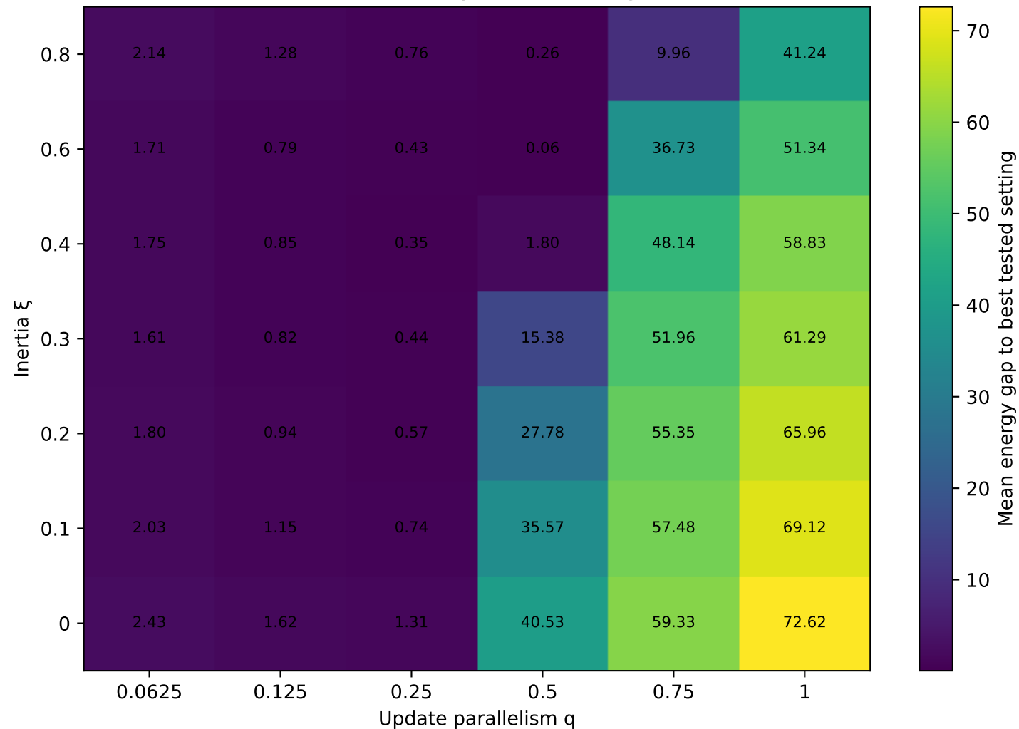
Dense ER Max-Cut: optimization degradation
