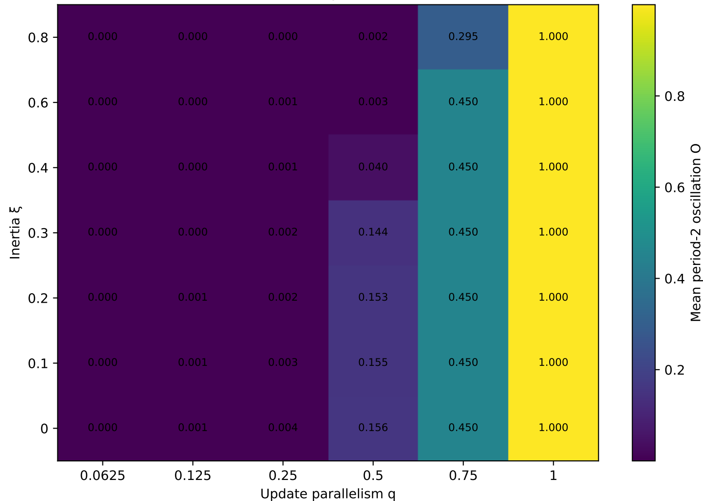
Dense ER Max-Cut: period-2 oscillation
