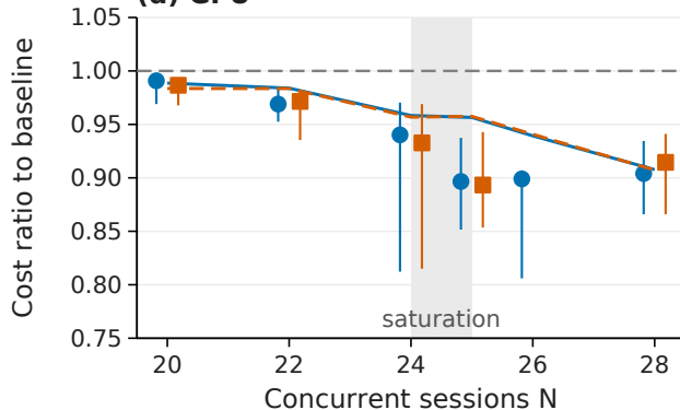
(d) GPU
