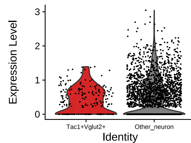
Il16
