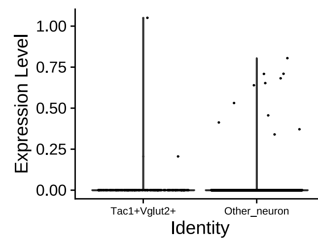
Calca
