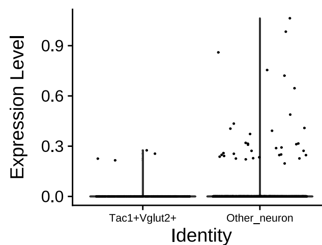
Trpv1
