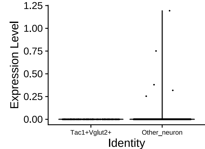
Scn10a
