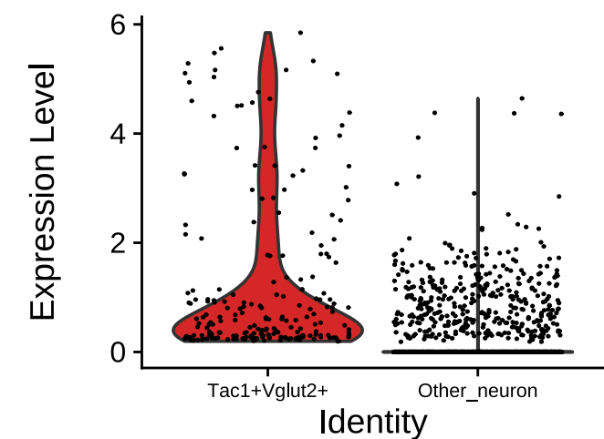
Scn10a
