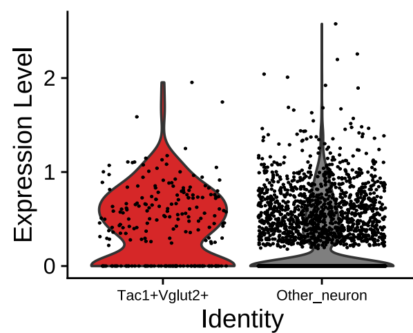
Arrb1
