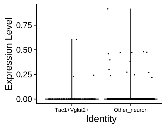
Btla
