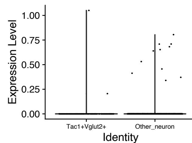
Calca
