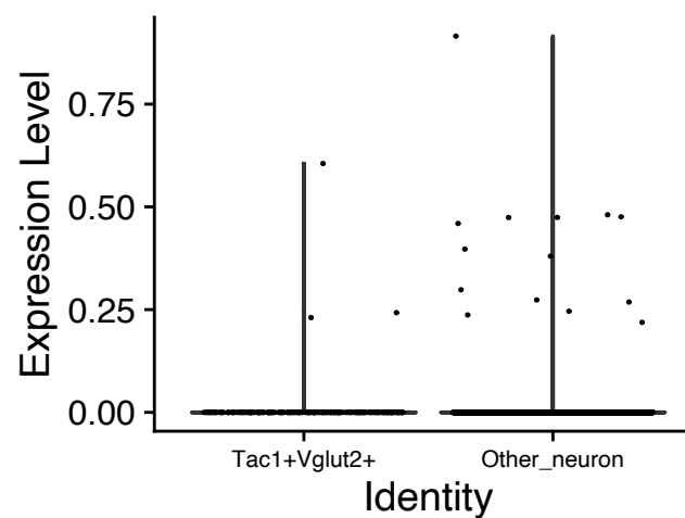
Btla
