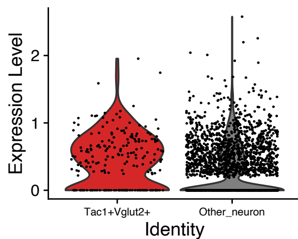
Arrb1
