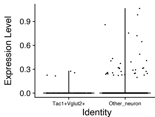
Trpv1
