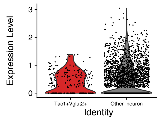
Il16
