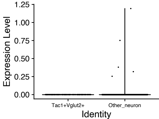
Scn10a
