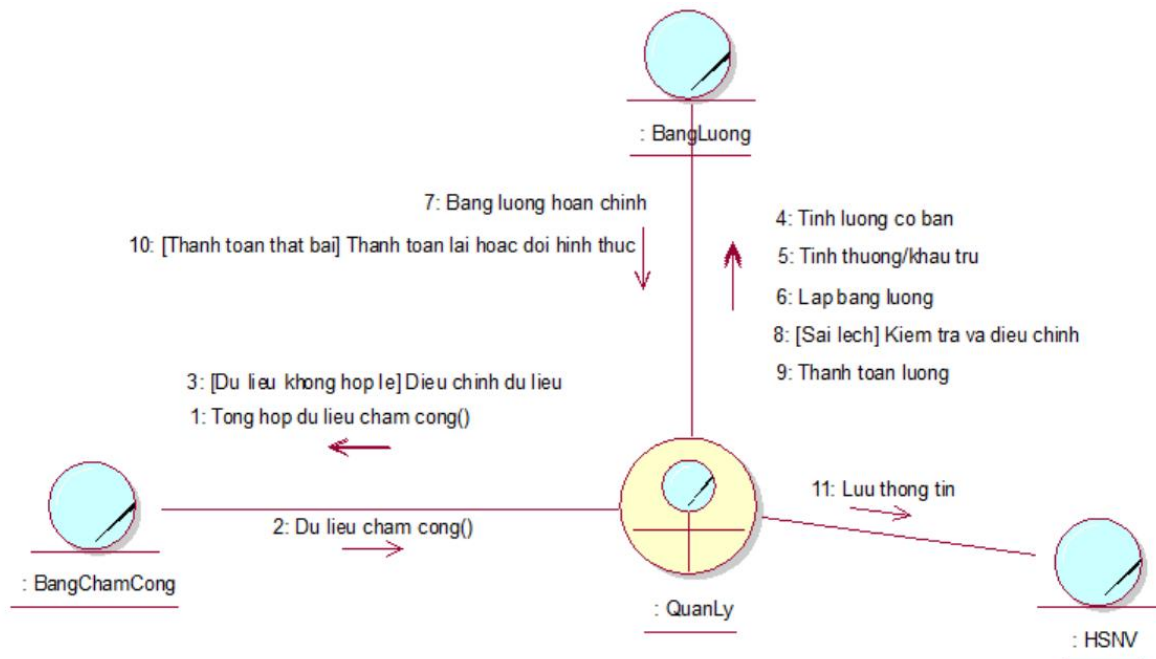
Hình 16: Sơ đồ cộng tác thanh toán lương
