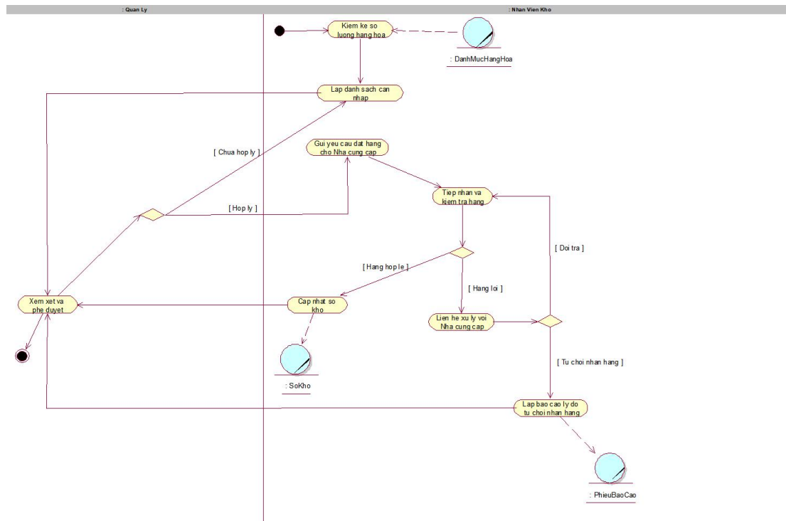
Hình 11: Sơ đồ hoạt động kiểm soát hàng hóa
