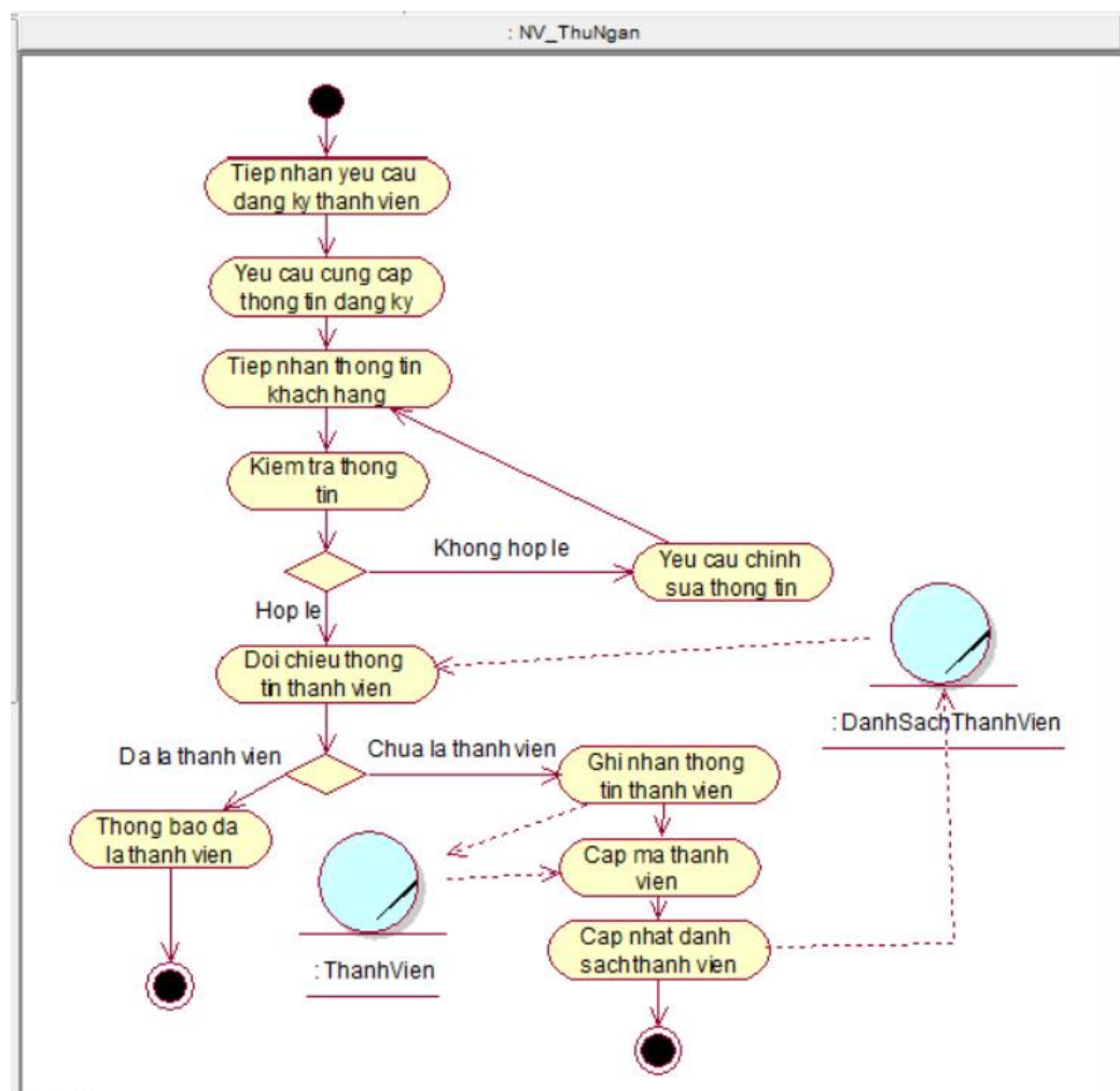
Hình 8: Sơ đồ hoạt động Đăng ký thành viên
