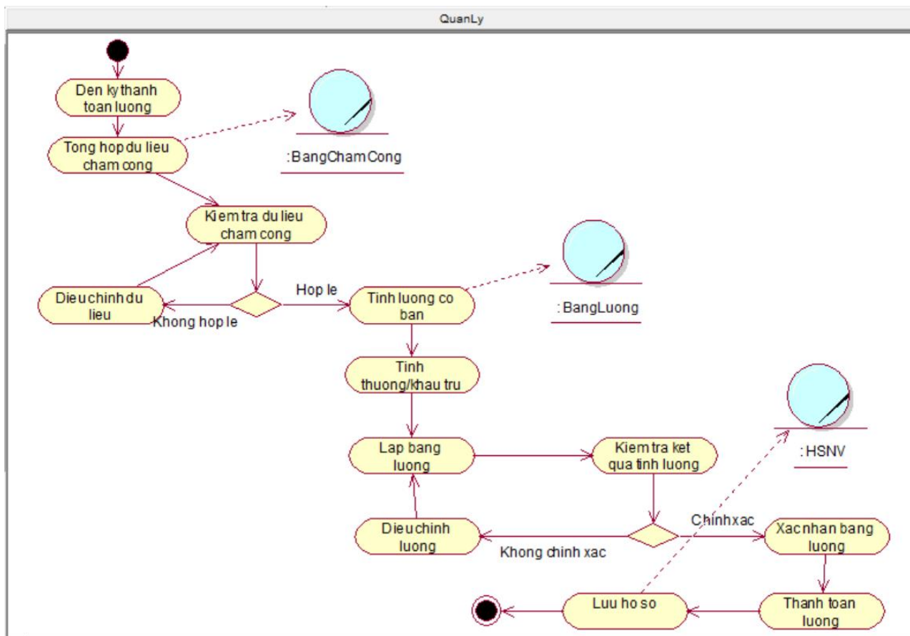
Hình 14: Sơ đồ hoạt động usecase thanh toán lương
