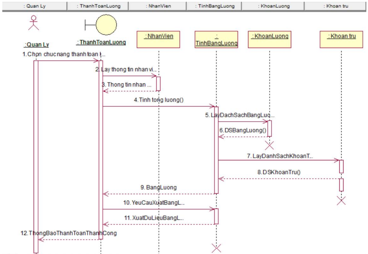
Hình 43: Sơ đồ tuần tự thiết kế hoạt động chức năng thanh toán lương
