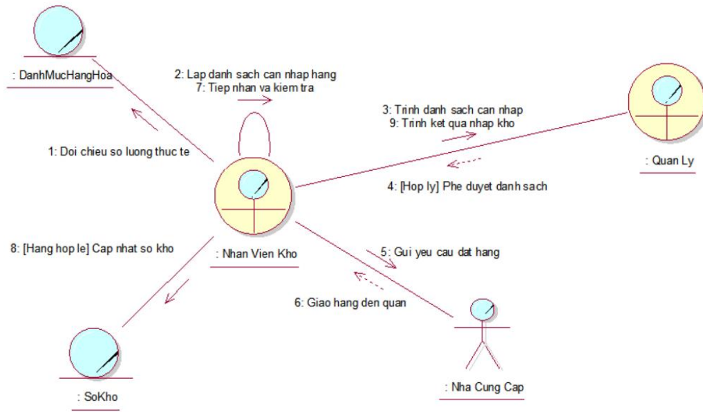
Hình 13: Sơ đồ cộng tác usecase kiểm soát hàng hóa
