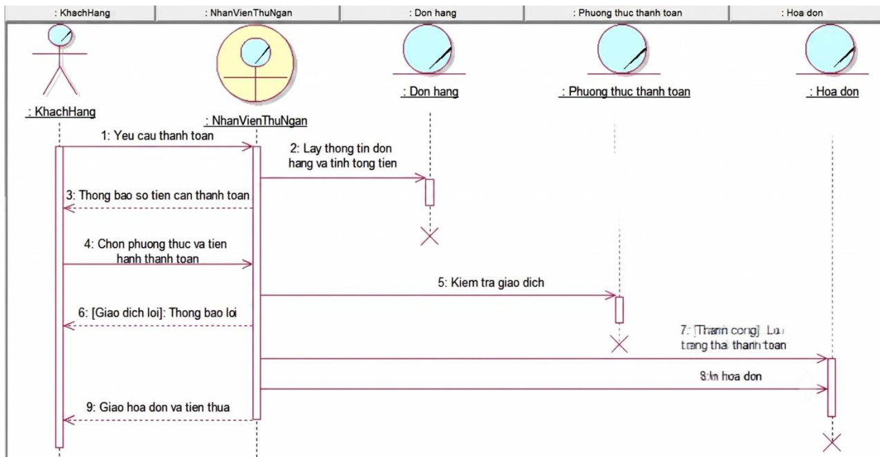
Hình 6: Sơ đồ tuần tự usecase thanh toán
