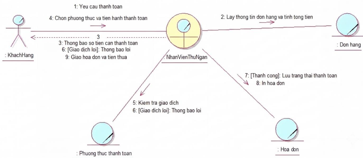
Hình 7: Sơ đồ cộng tác usecase thanh toán
