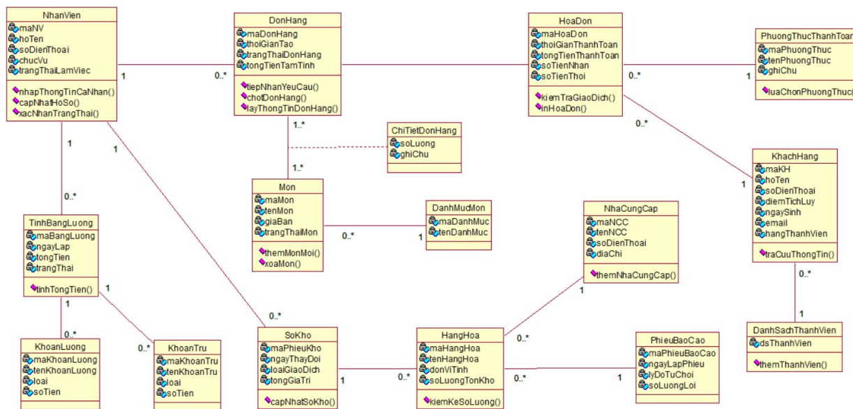
Hình 18: Sơ đồ lớp phân tích hệ thống quản lý quán cà phê
