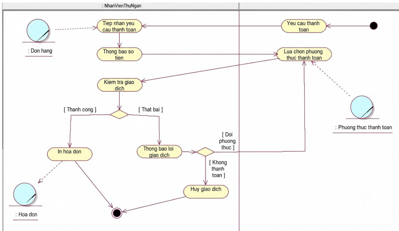
Hình 5: Sơ đồ hoạt động usecase thanh toán
