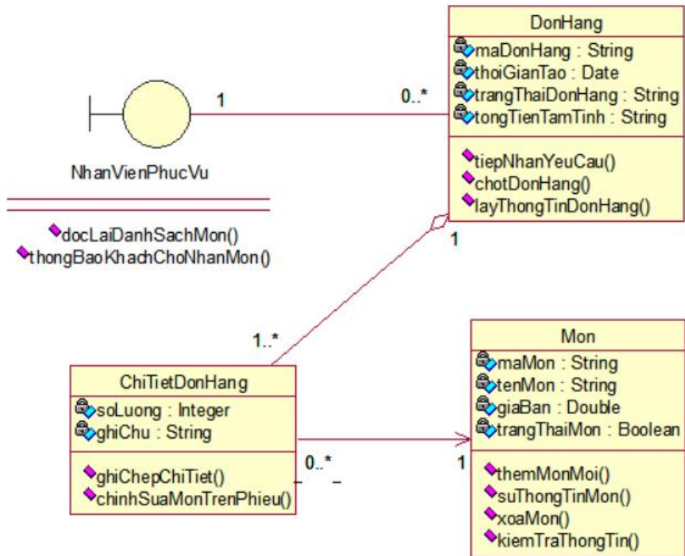
Hình 34: Sơ đồ lớp mức thiết kế chức năng Gọi món
