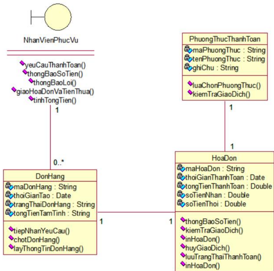
Hình 36: Sơ đồ lớp mức thiết kế chức năng Thanh toán
