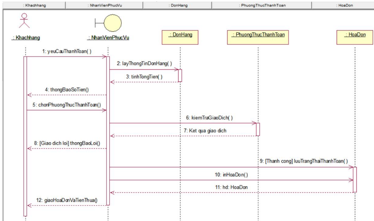
Hình 37: Sơ đồ tuần tự thiết kế hoạt động chức năng Thanh toán
