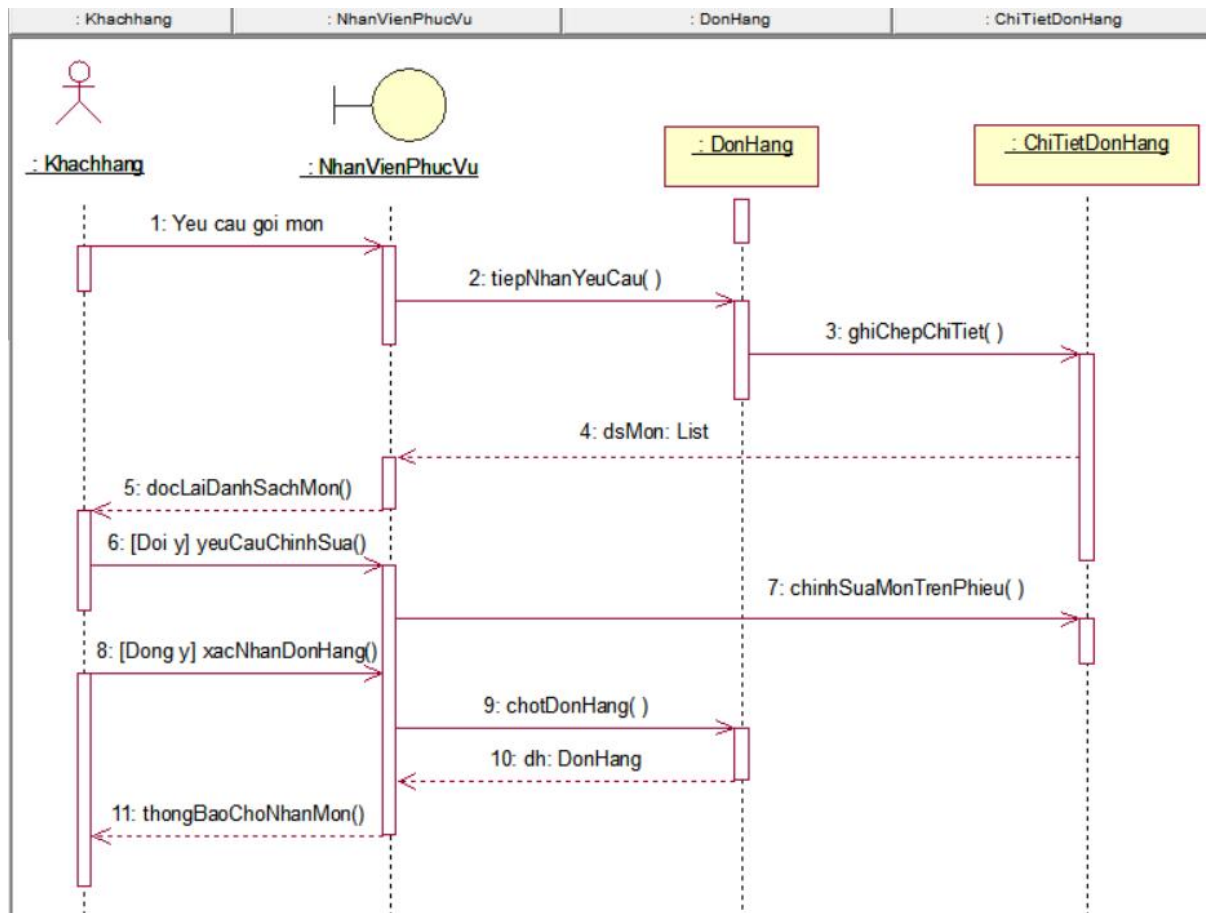
Hình 35: Sơ đồ tuần tự thiết kế hoạt động chức năng Gọi món
