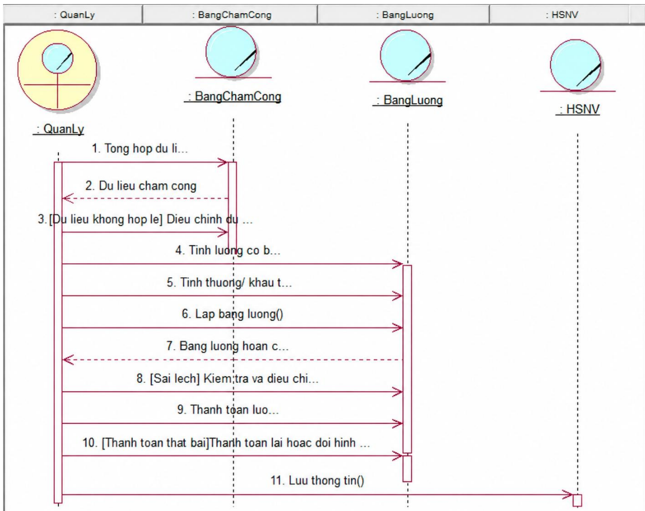
Hình 15: Sơ đồ tuần tự thanh toán lương
