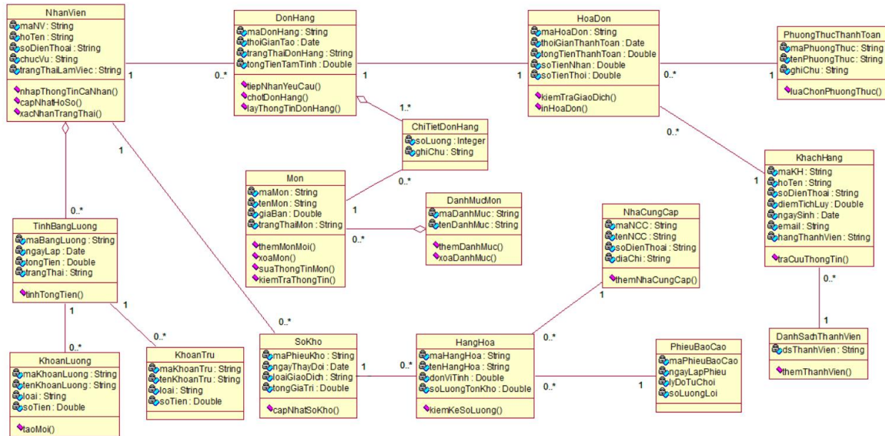
Hình 33: Sơ đồ lớp mức thiết kế hệ thống quản lý cà phê
