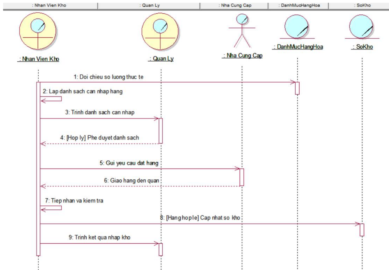
Hình 12: Sơ đồ tuần tự kiểm soát hàng hóa
