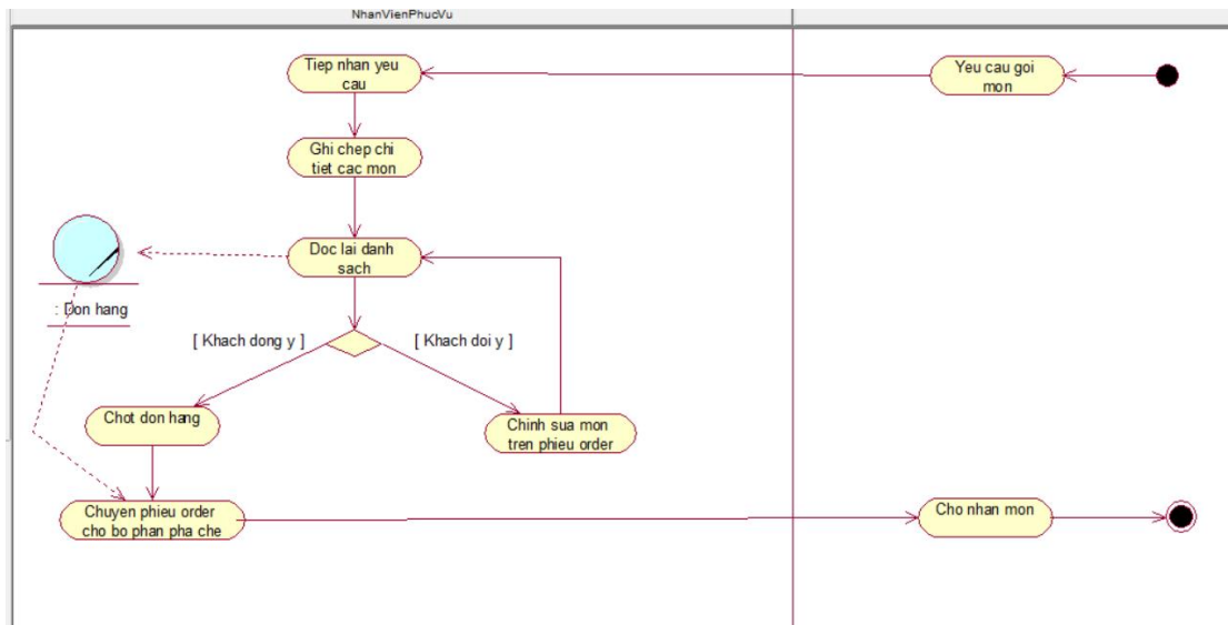
Hình 2: Sơ đồ hoạt động usecase gọi món
