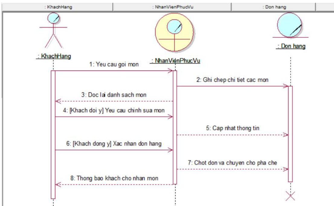
Hình 3: Sơ đồ tương tác usecase gọi món
