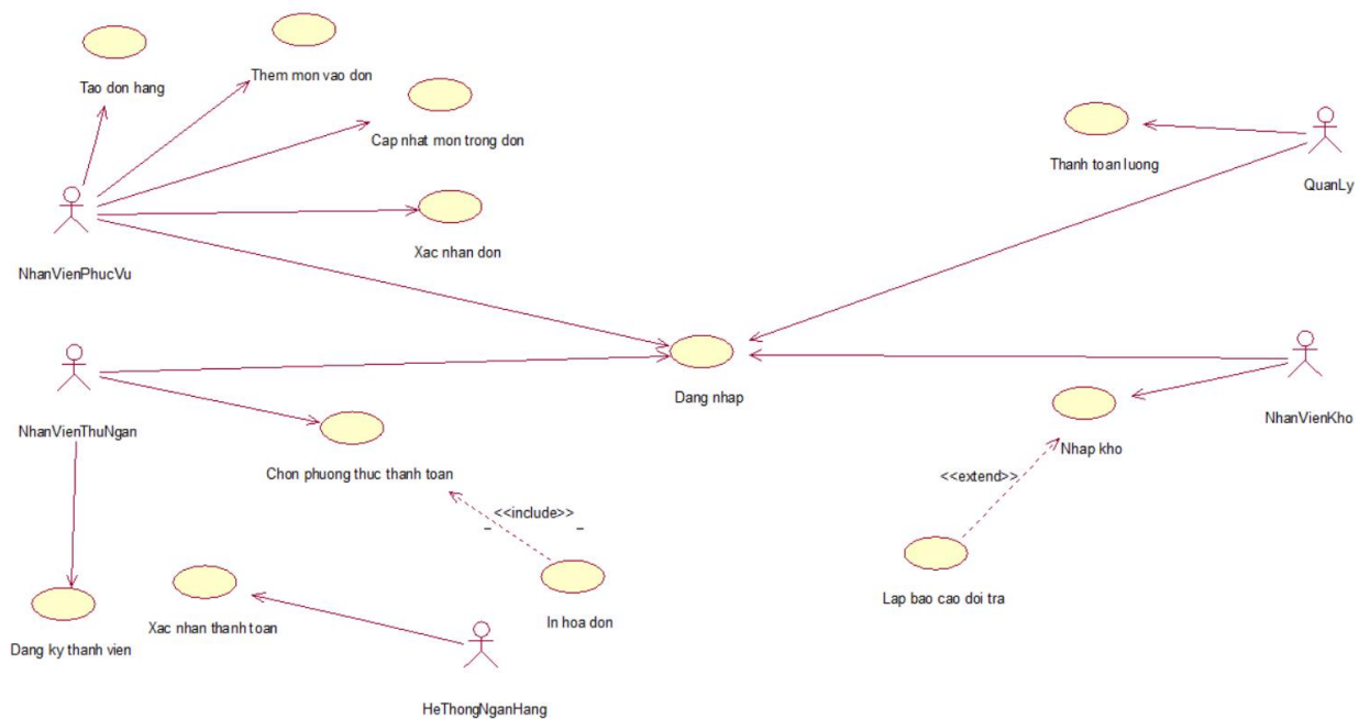
Hình 17: Sơ đồ usecase hệ thống quản lý quán cà phê
