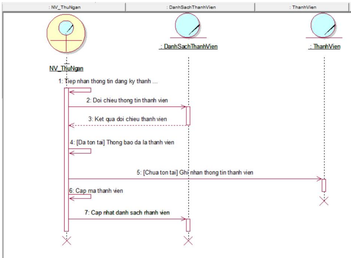
Hình 9: Sơ đồ tuần tự usecase Đăng ký thành viên
