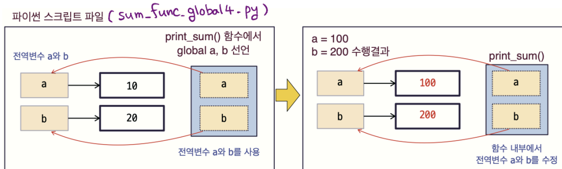
[그림 5-9] 명시적 global 선언을 통하여 함수 내에서 전역변수 a, b를 사용하는 과정
