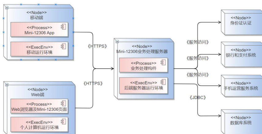
图 1. “Mini-12306”软件的部署图
