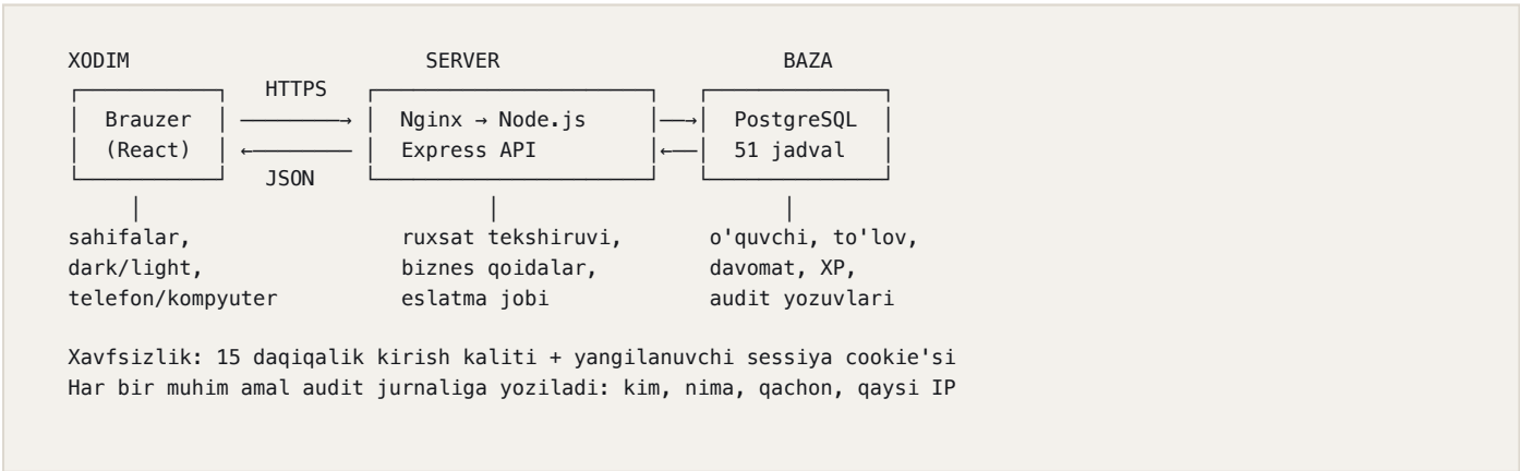
SXEMA 2 – QATLAMLAR
