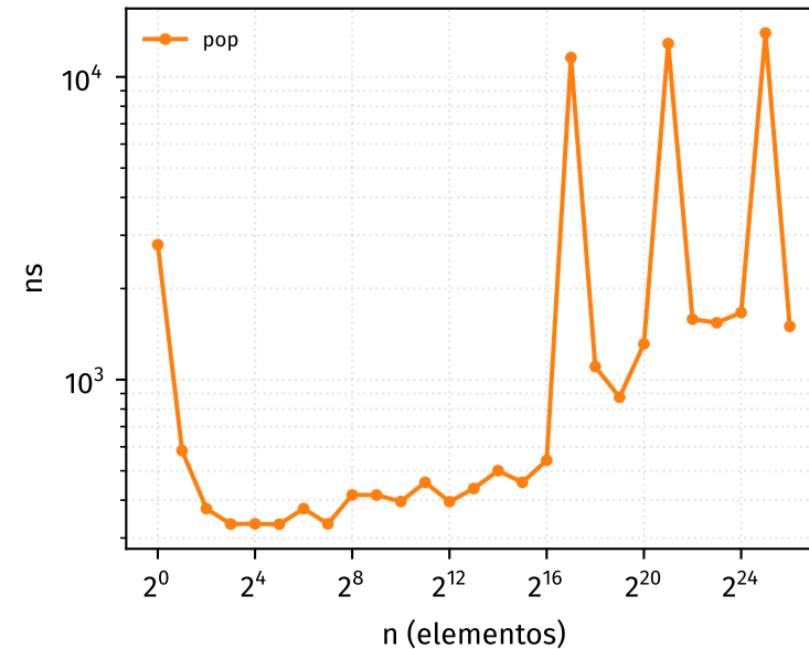
pop
