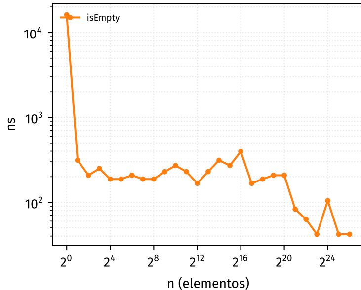
isEmpty
