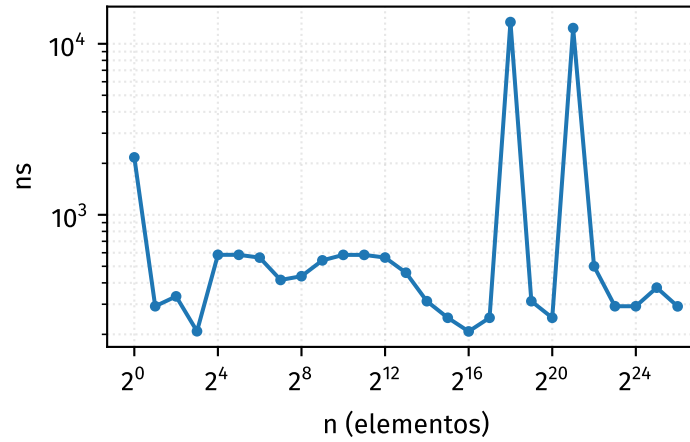
addAfter
