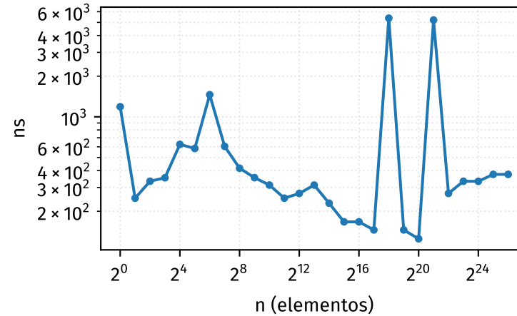
addAfter
