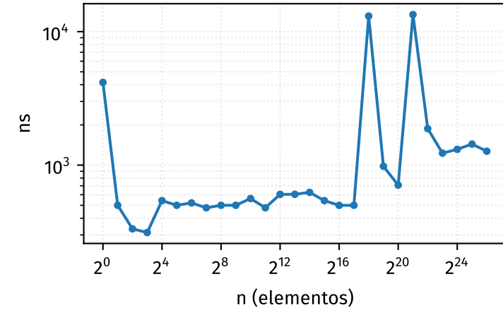
popBack
