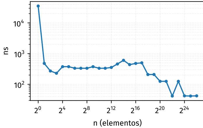
isEmpty
