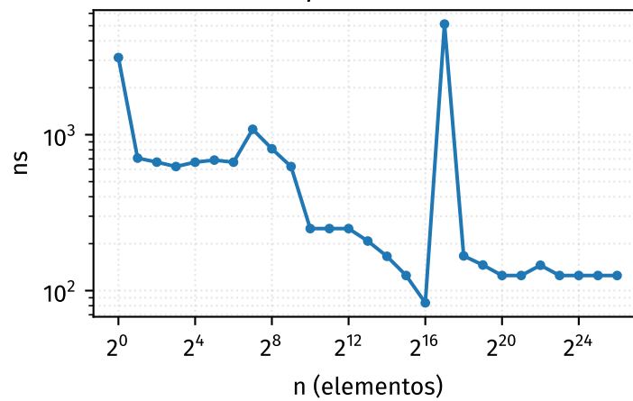
popFront
