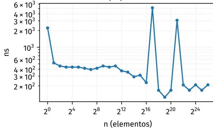
addAfter
