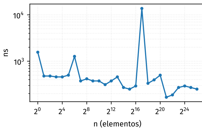
addAfter
