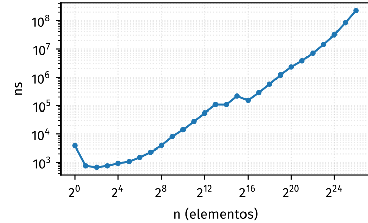
popBack
