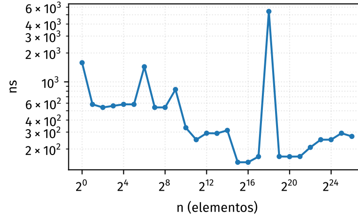
addAfter
