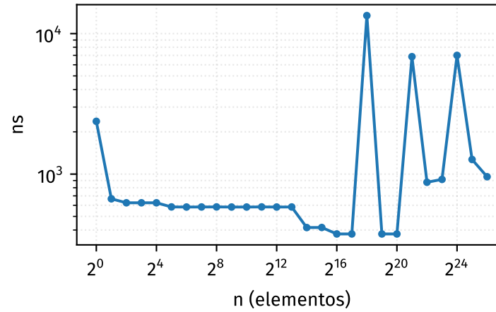
addAfter
