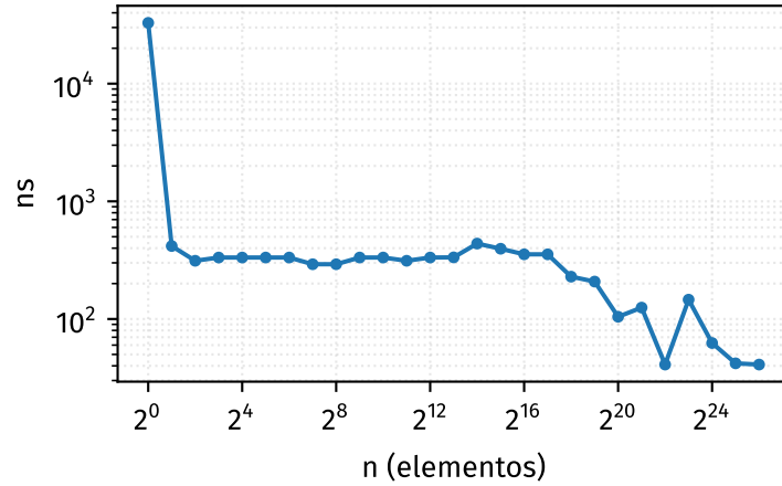
isEmpty
