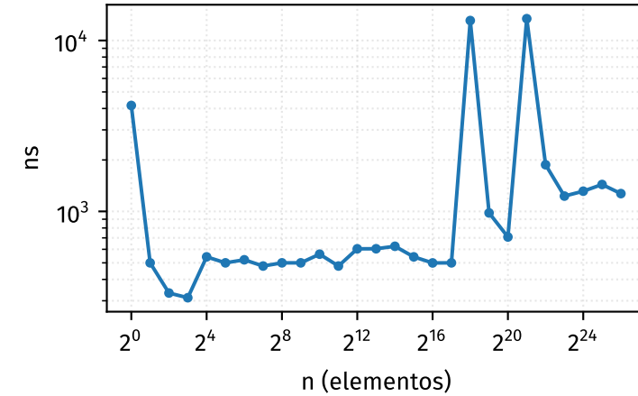
popBack
