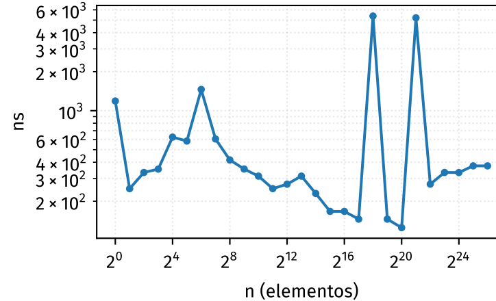
addAfter
