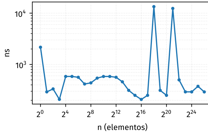
popFront
