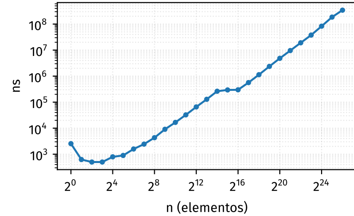
popBack
