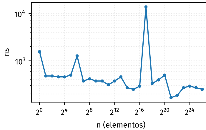
addAfter
