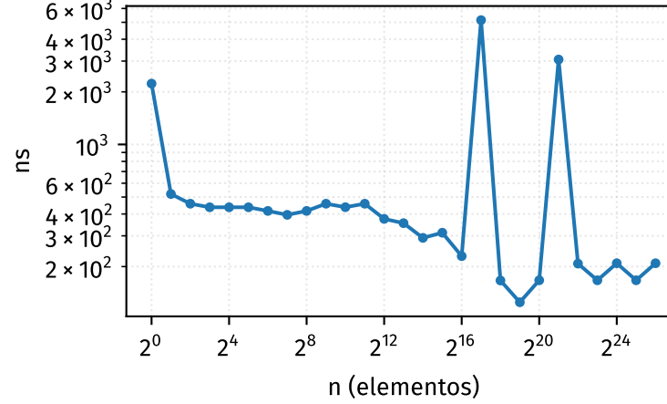
addAfter
