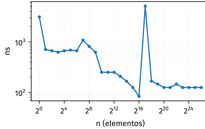
popFront
