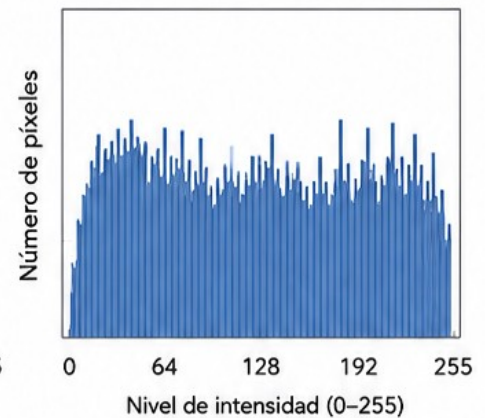
Histograma ecualizado
