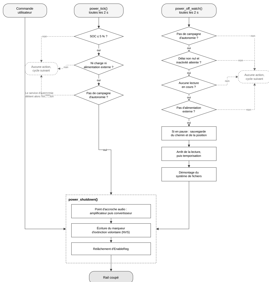
Figure 5.5 – Séquence d'extinction. Les trois voies d'entrée convergent vers un corps commun qui descend la pile de haut en bas. Les branches en pointillé rendent la main au cycle suivant sans agir.
