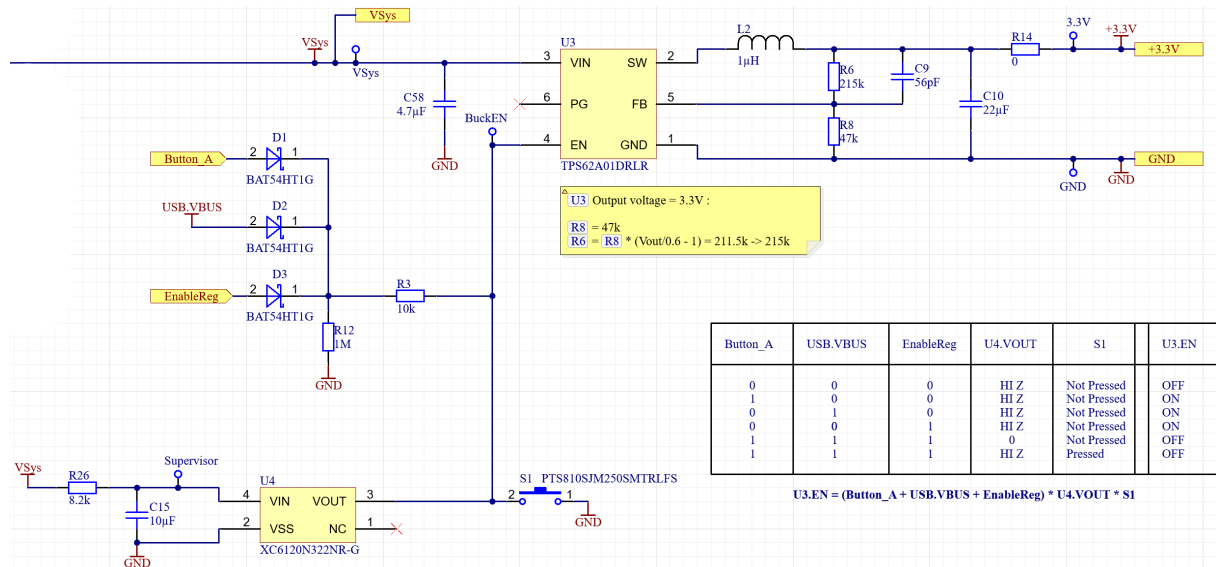
Figure 4.2 – Extrait du schéma, logique d'activation du convertisseur et superviseur de tension
