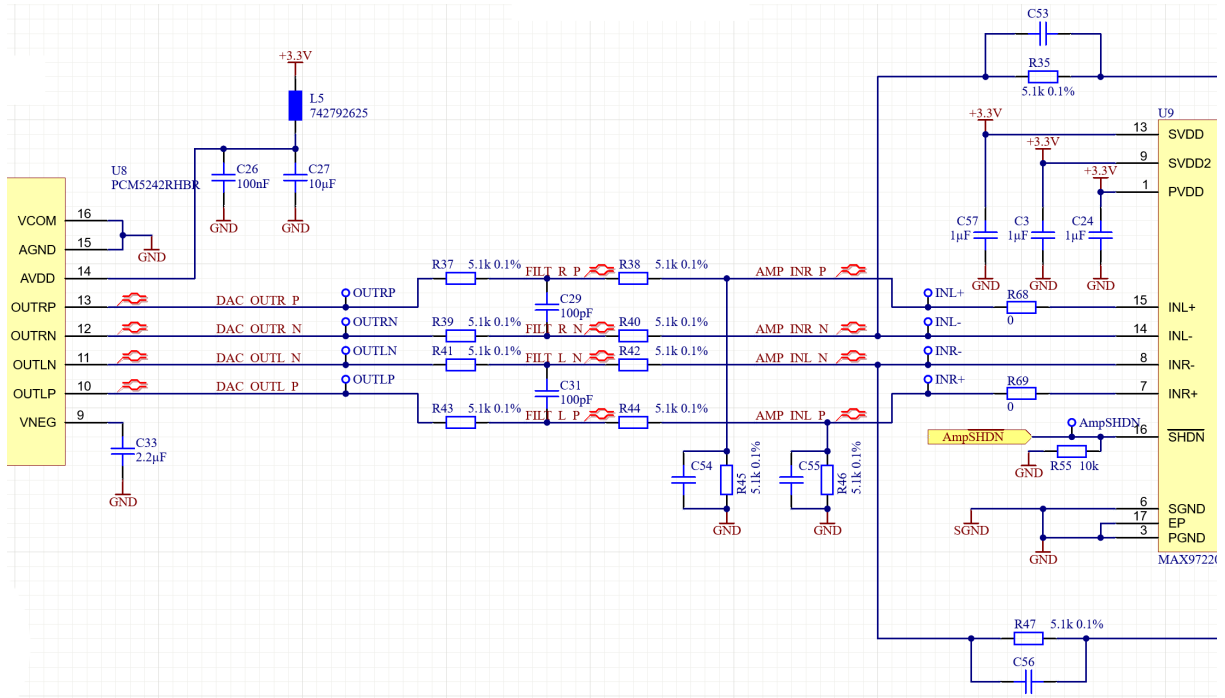
Figure 4.3 – Extrait du schéma, sorties différentielles du convertisseur, filtre passif et entrées de l'amplificateur
