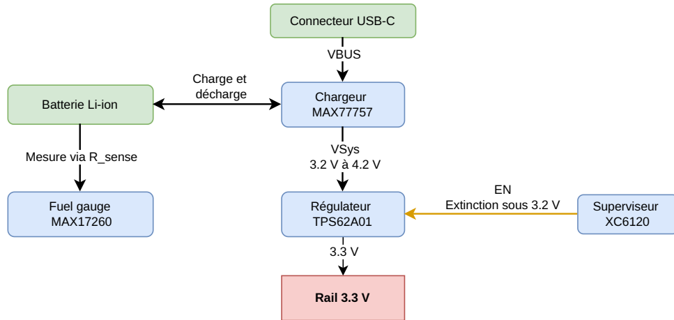
Figure 4.1 – Arbre d'alimentation, de l'entrée USB au rail logique
