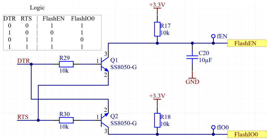
Figure 4.4 – Extrait du schéma, circuit de passage automatique en mode programmation
