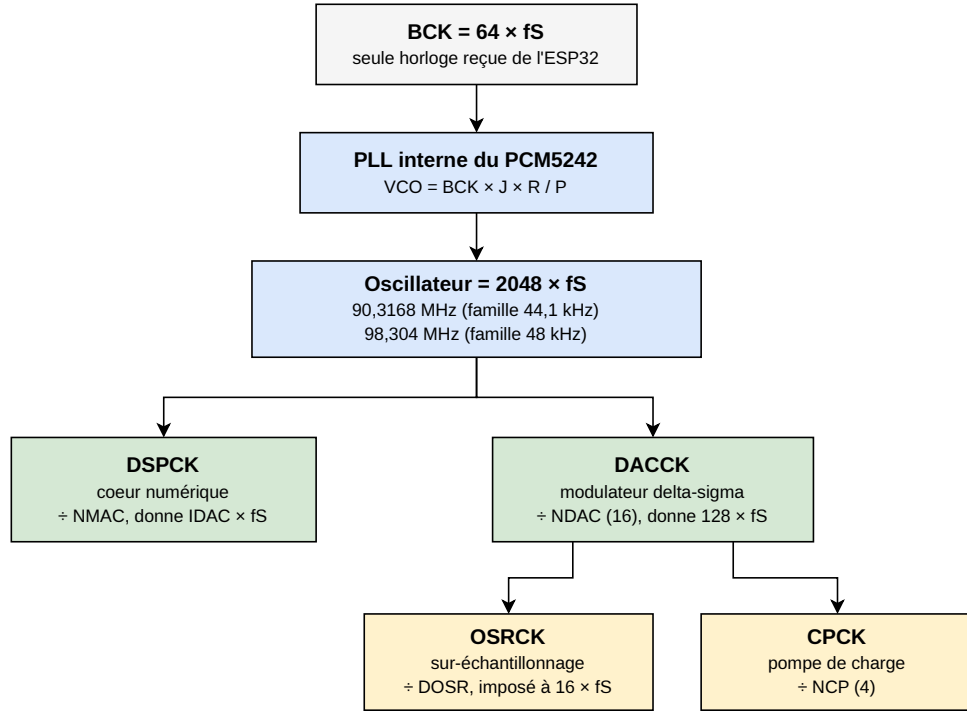
Figure 5.2 – Arbre d'horloge interne du PCM5242. La boucle à verrouillage de phase porte l'horloge de bit à un oscillateur valant 2048 fois la fréquence d'échantillonnage, dont dérivent l'horloge du cœur numérique et celle du modulateur, cette dernière alimentant à son tour le filtre de sur-échantillonnage et la pompe de charge.
