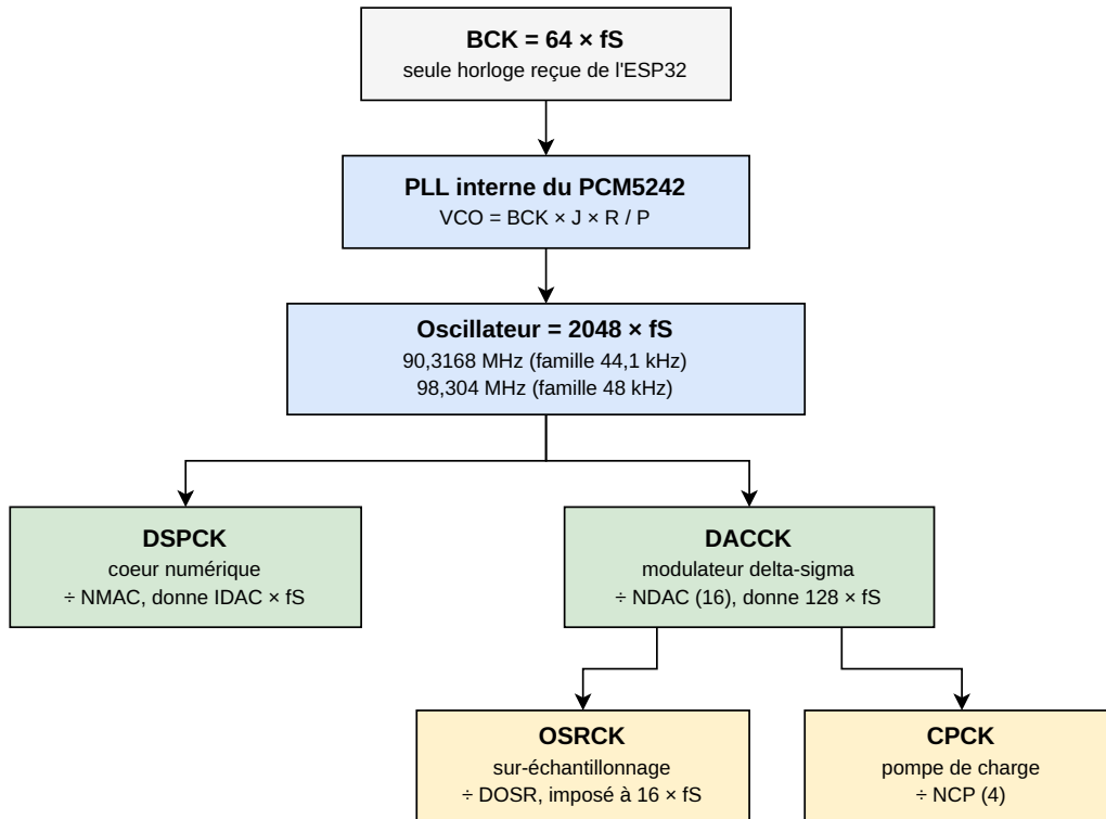
Figure 5.4 – Arbre d'horloge interne du PCM5242. La boucle à verrouillage de phase porte l'horloge de bit à un oscillateur valant 2048 fois la fréquence d'échantillonnage, dont dérivent l'horloge du cœur numérique et celle du modulateur, cette dernière alimentant à son tour le filtre de sur-échantillonnage et la pompe de charge.
