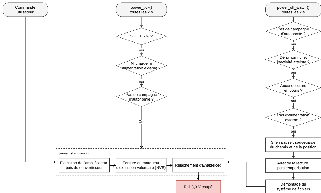
Figure 5.5 – Séquence d'extinction. Les trois voies d'entrée convergent vers un corps commun. Une réponse négative à l'une des gardes rend la main au cycle suivant sans action.
