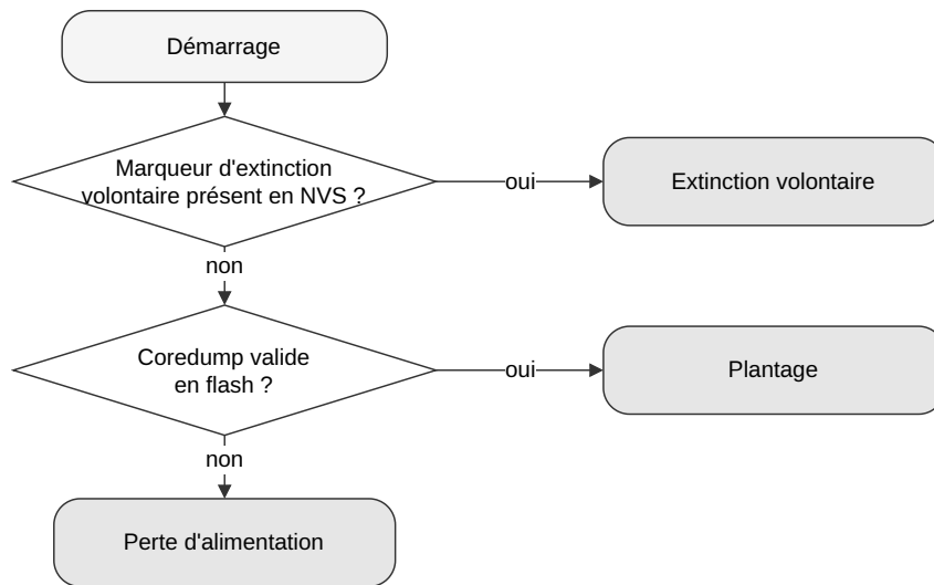
Figure 5.6 – Reconstitution de la fin de la session précédente. Les deux témoins sont exclusifs, un plantage n’atteignant jamais le code qui écrit le marqueur.
