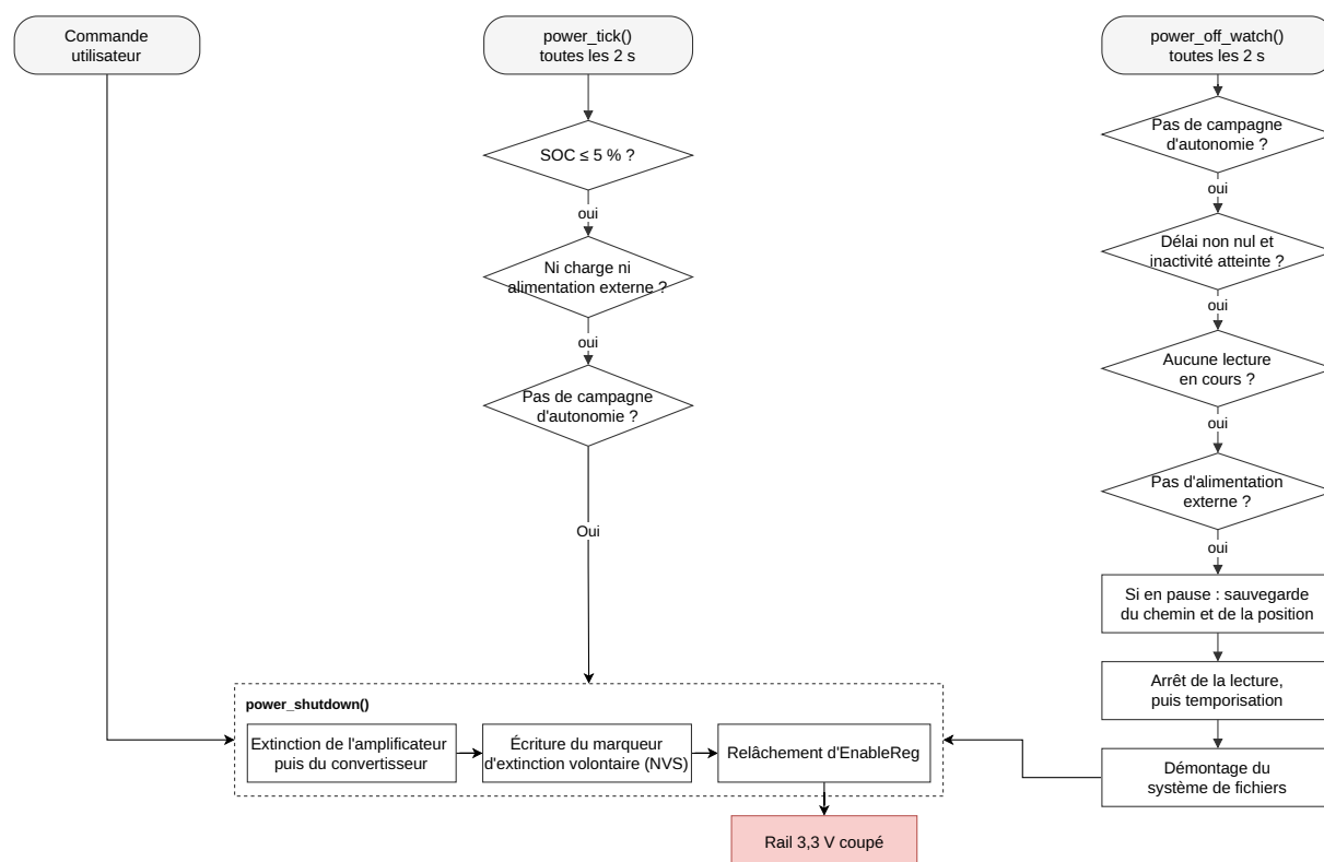
Figure 5.5 — Séquence d'extinction. Les trois voies d'entrée convergent vers un corps commun qui descend la pile de haut en bas. Les branches en pointillé rendent la main au cycle suivant sans agir.
