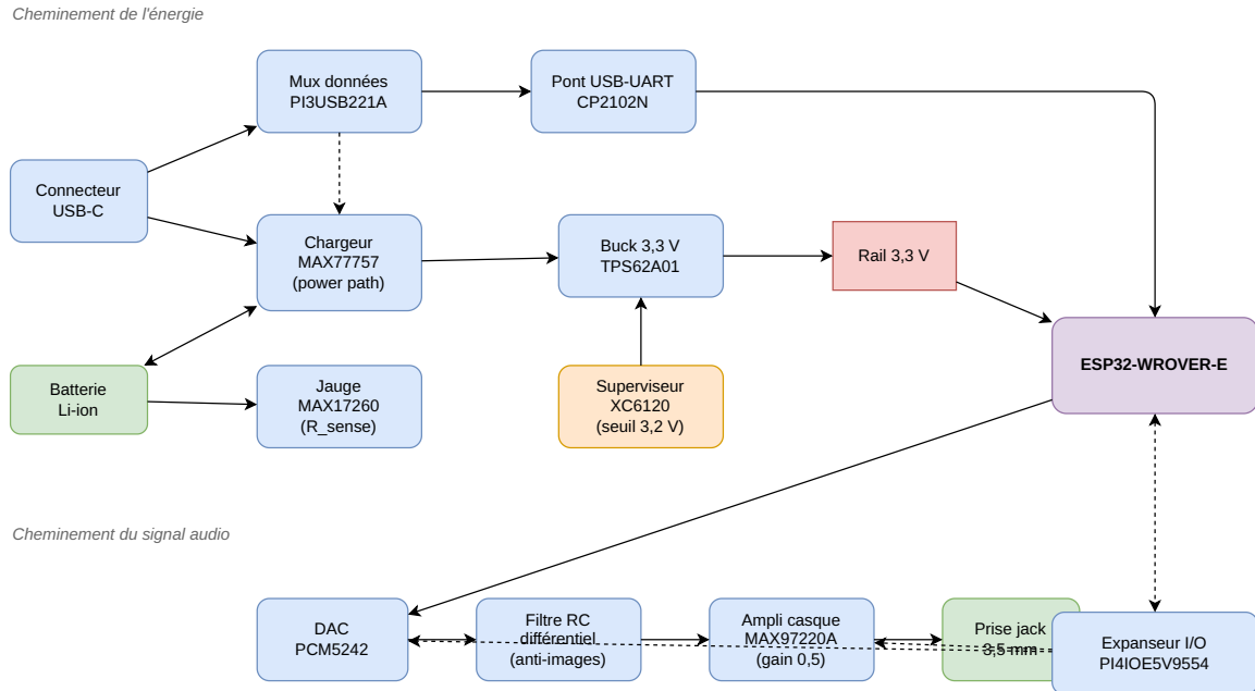
Figure 4.1 – Architecture électrique du lecteur, cheminement de l'énergie et du signal audio
