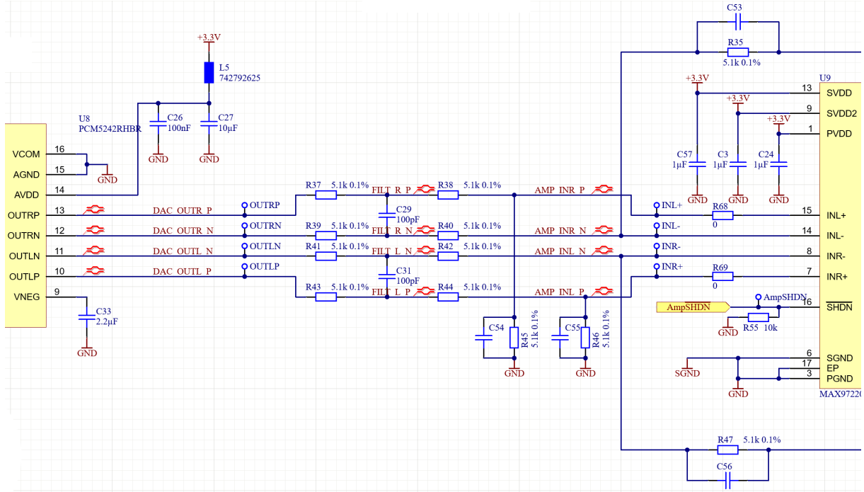
Figure 4.4 – Extrait du schéma, sorties différentielles du convertisseur, filtre passif et entrées de l'amplificateur
