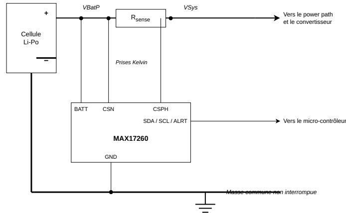
Figure 4.1 – Mesure de courant côté haut, position de la résistance de mesure entre la cellule et le nœud système
