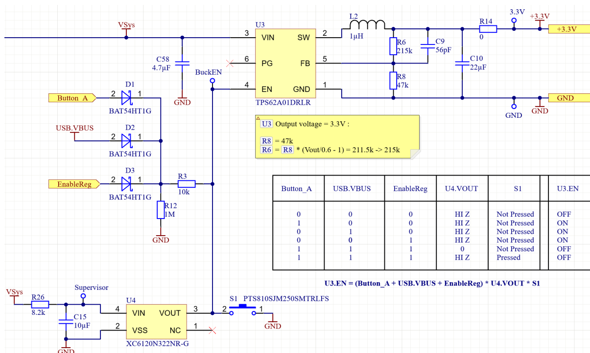
Figure 4.3 – Extrait du schéma, logique d'activation du convertisseur et superviseur de tension
