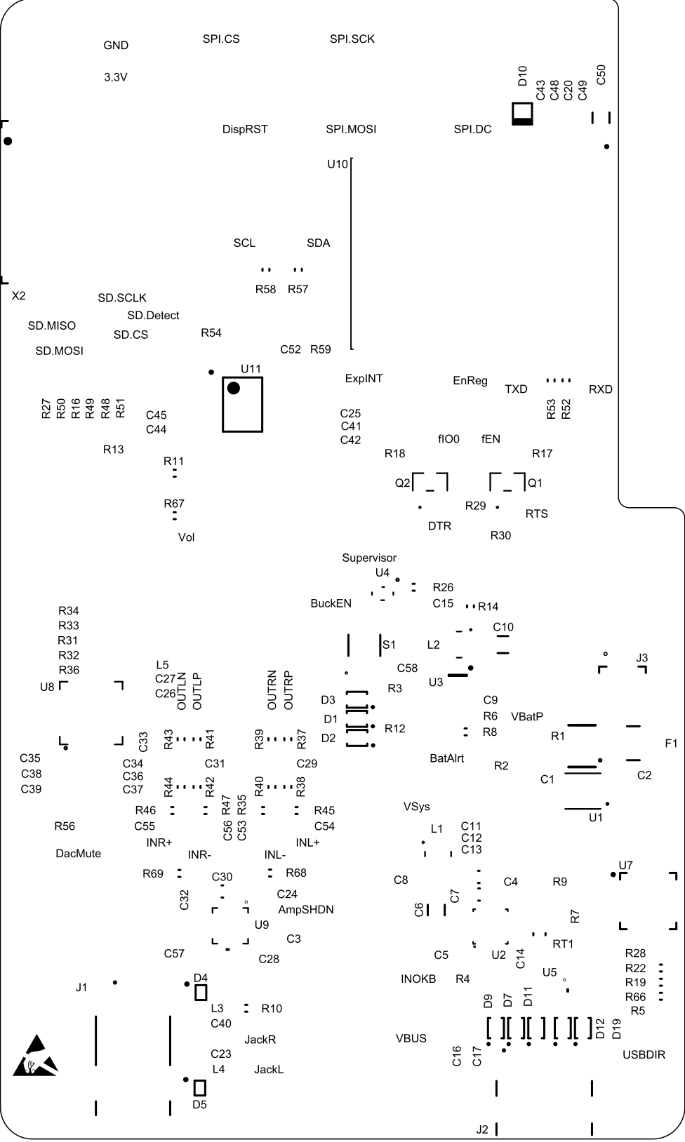
Top Overlay (Scale 2:1)
