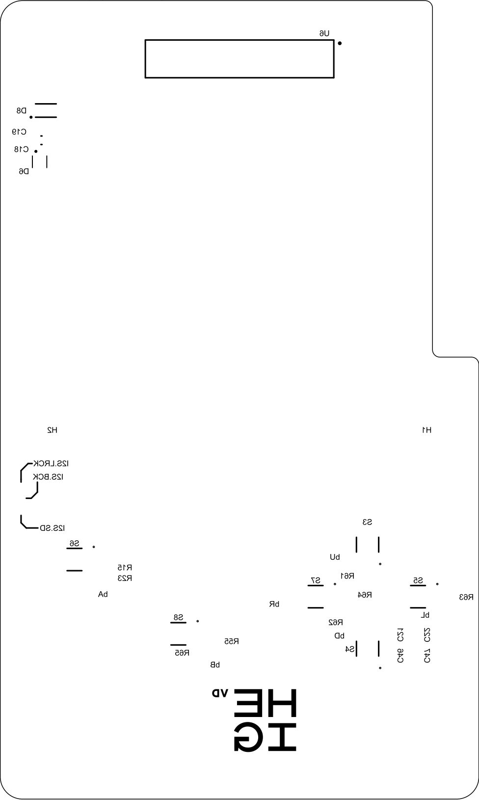
Bottom Overlay (Scale 2:1)
