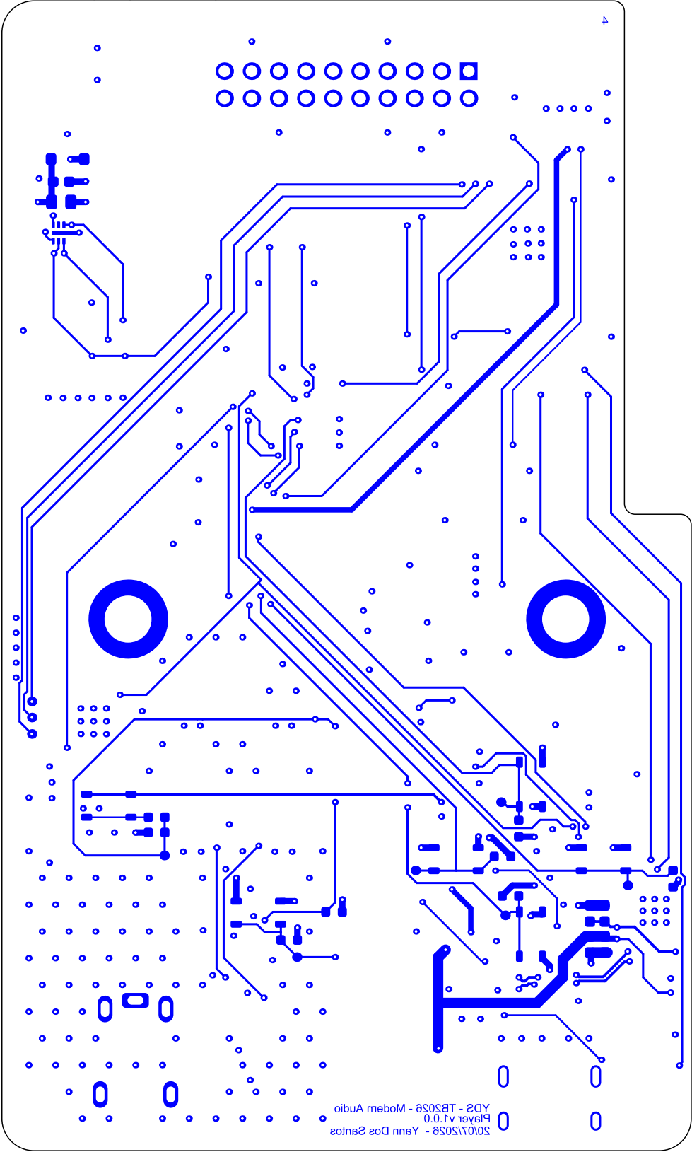
Bottom Layer (Scale 2:1)
