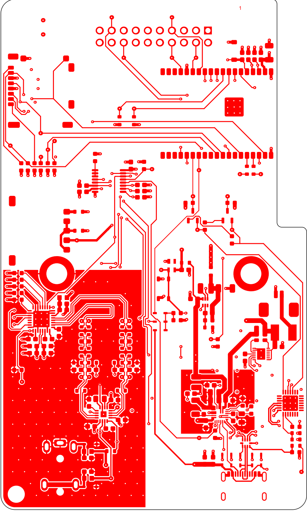
Top Layer (Scale 2:1)
