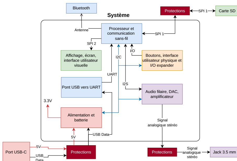
Figure 3.2 – Analyse fonctionnelle - Niveau 2
